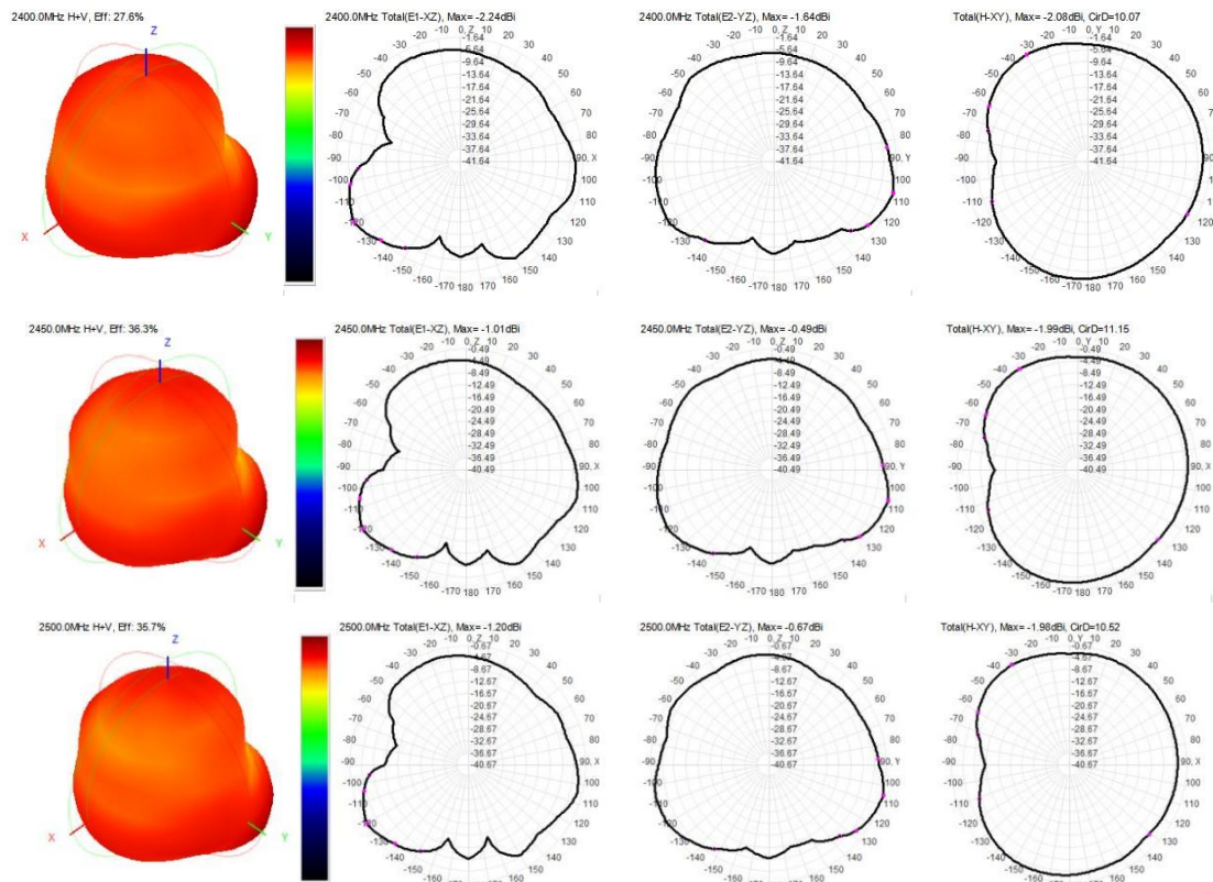
图 9 天线场型图
