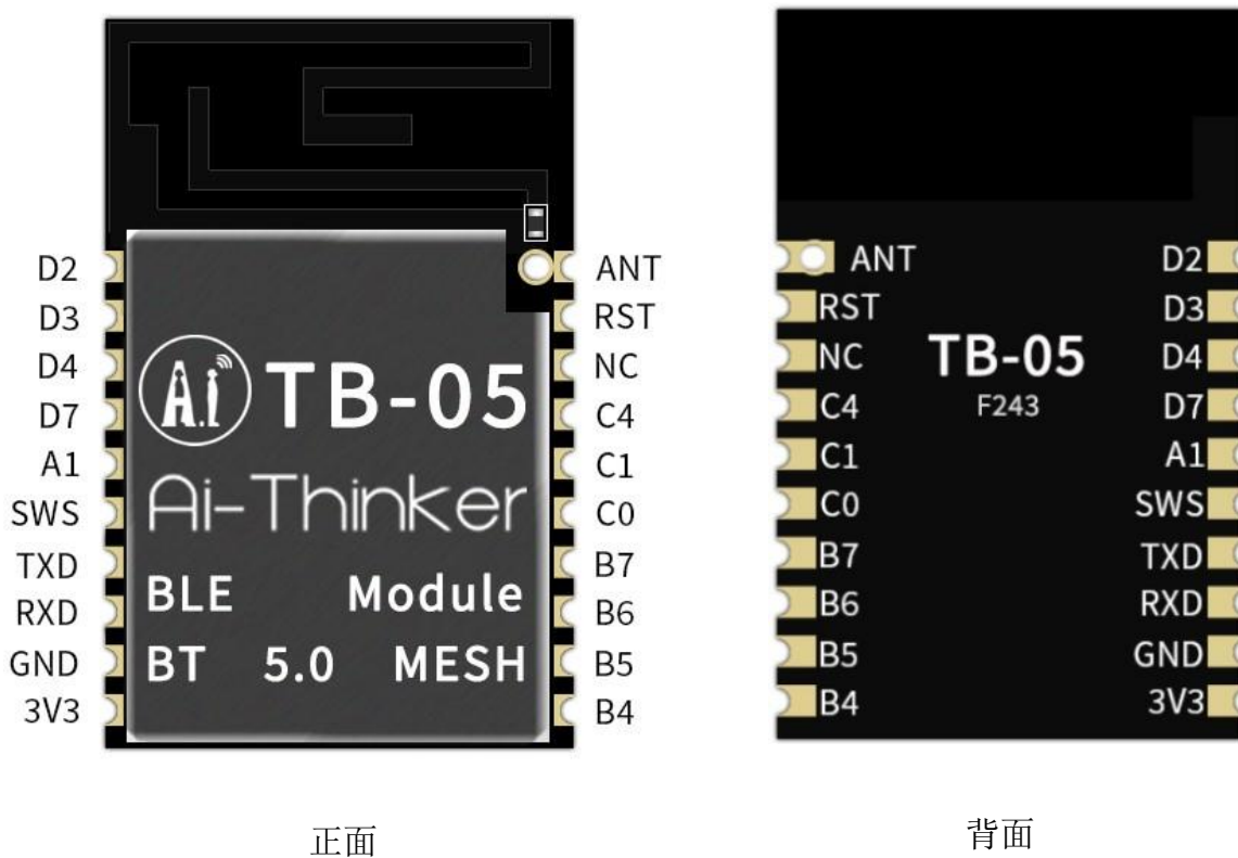
图 5 管脚顶视图
