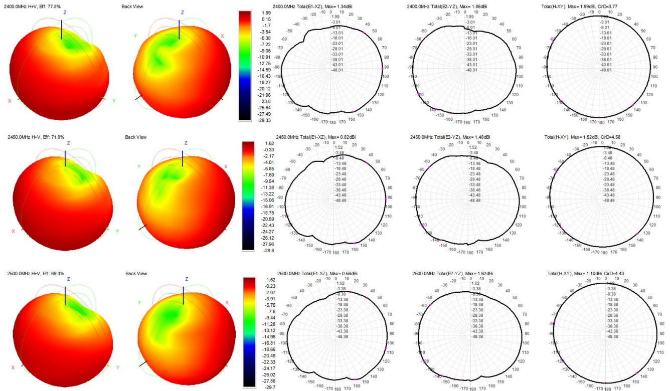
图 9 天线场型图
