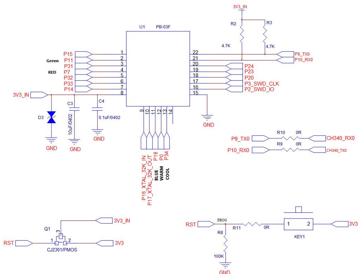
图 10 应用电路图
