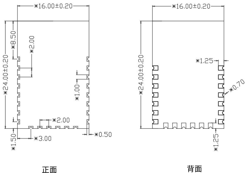
图 4 模组尺寸图
