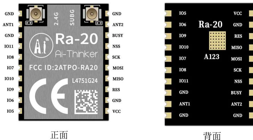
图 5 管脚示意图
