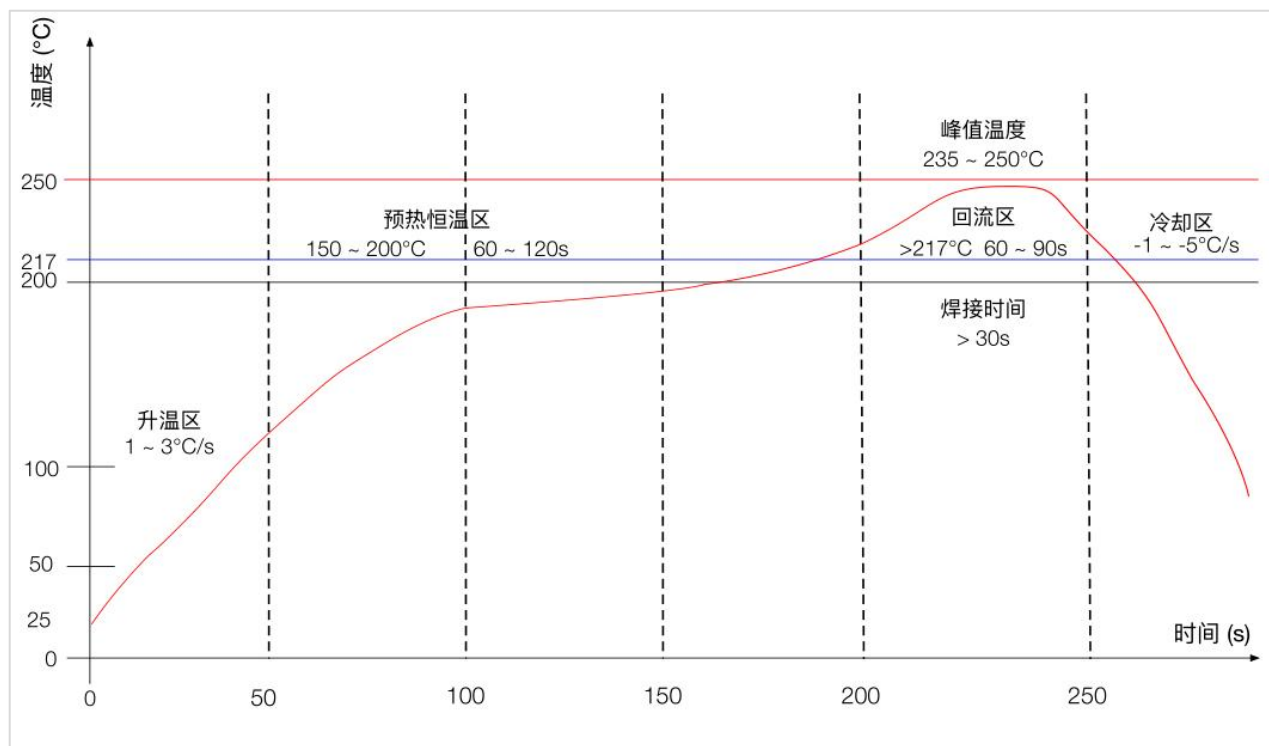
图 11 回流焊曲线
