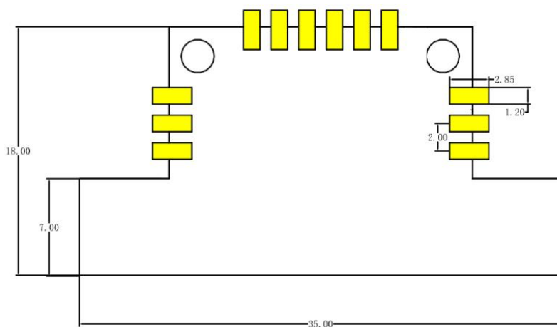
图 9 推荐 PCB 封装尺寸（单位：mm）
