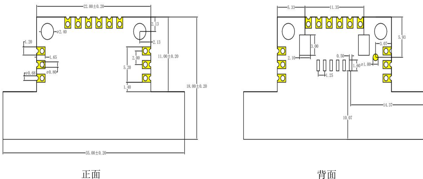
图 5 尺寸图（单位：mm）
