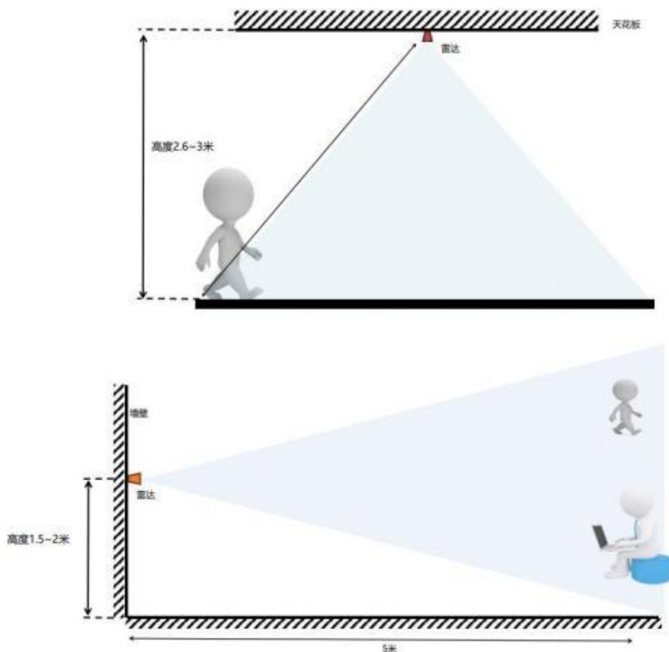
图 1 Rd-01 使用方式
