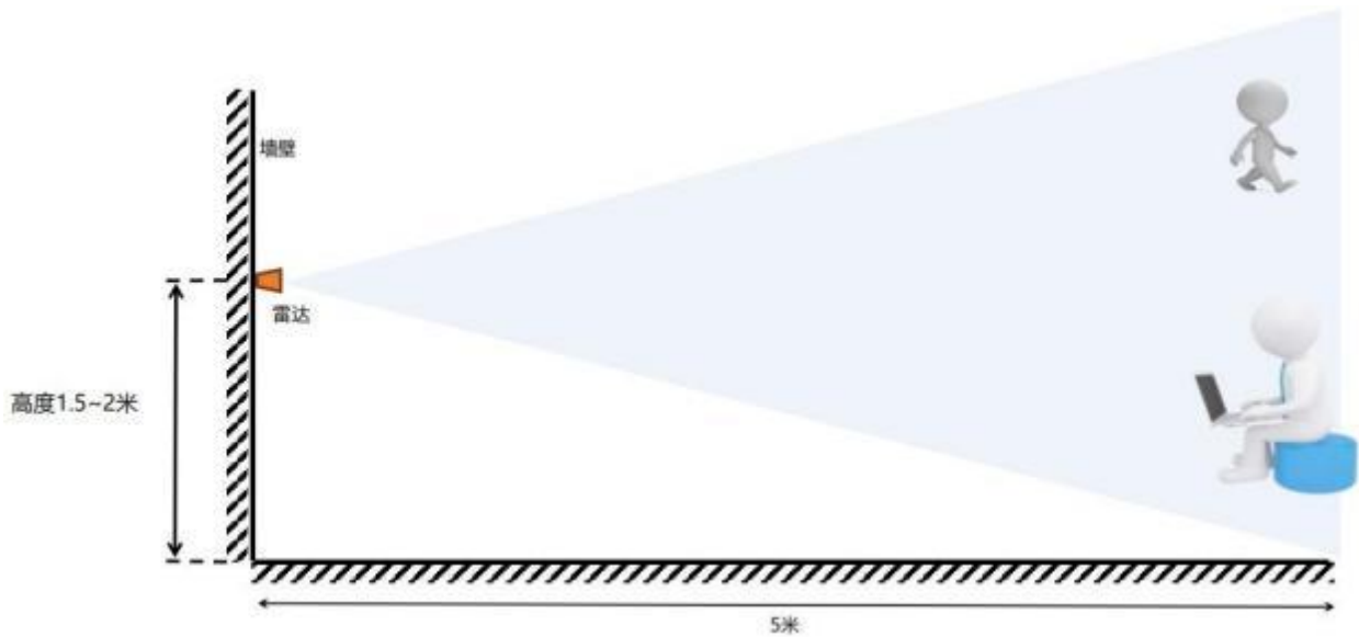
图 10 挂壁安装示意图
