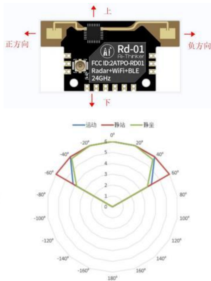
图 11 挂壁安装探测范围示意图
