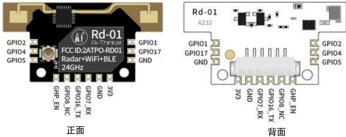
图 4 管脚示意图
