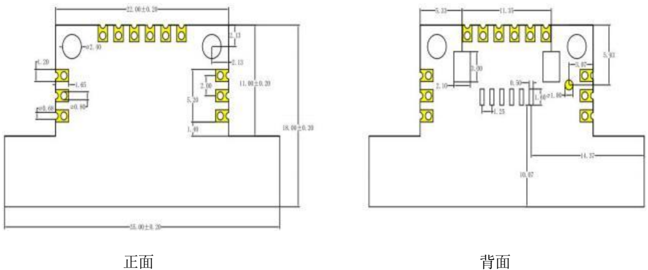
图 3 尺寸图
