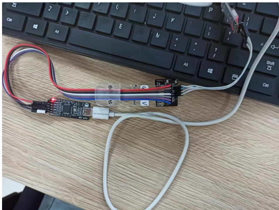
图 1.1 DAP 烧录接线
