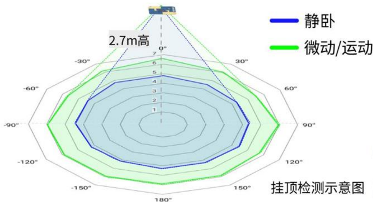
图 17 挂顶安装感应范围
