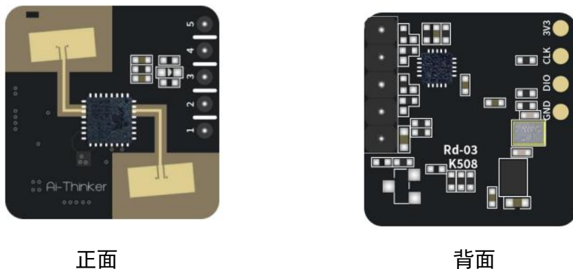
图 1 管脚示意图
