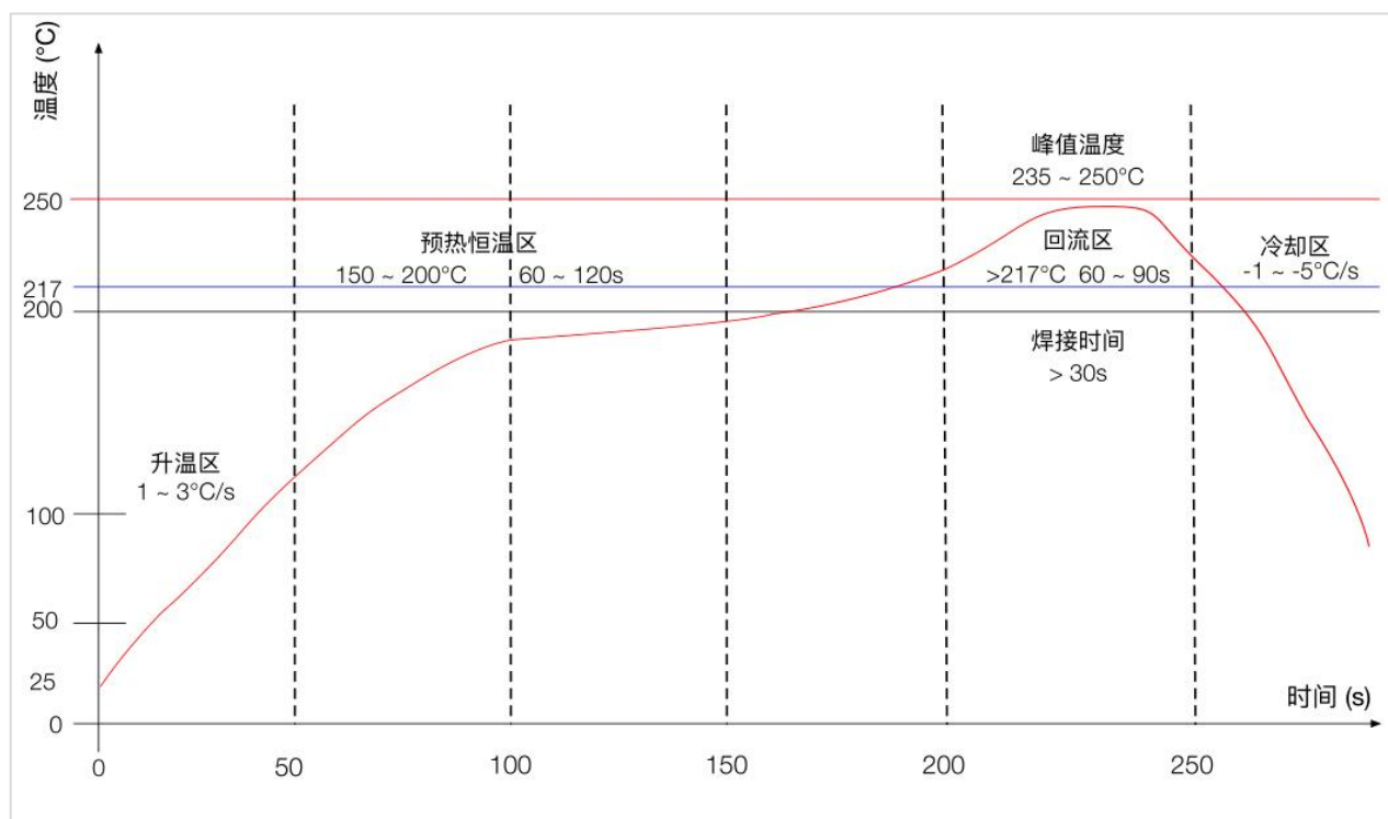
图 13 回流焊曲线
