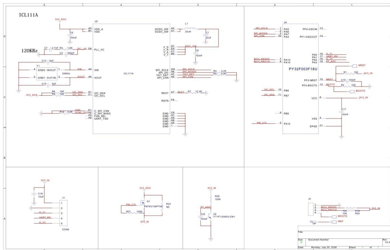
图 5 原理图
