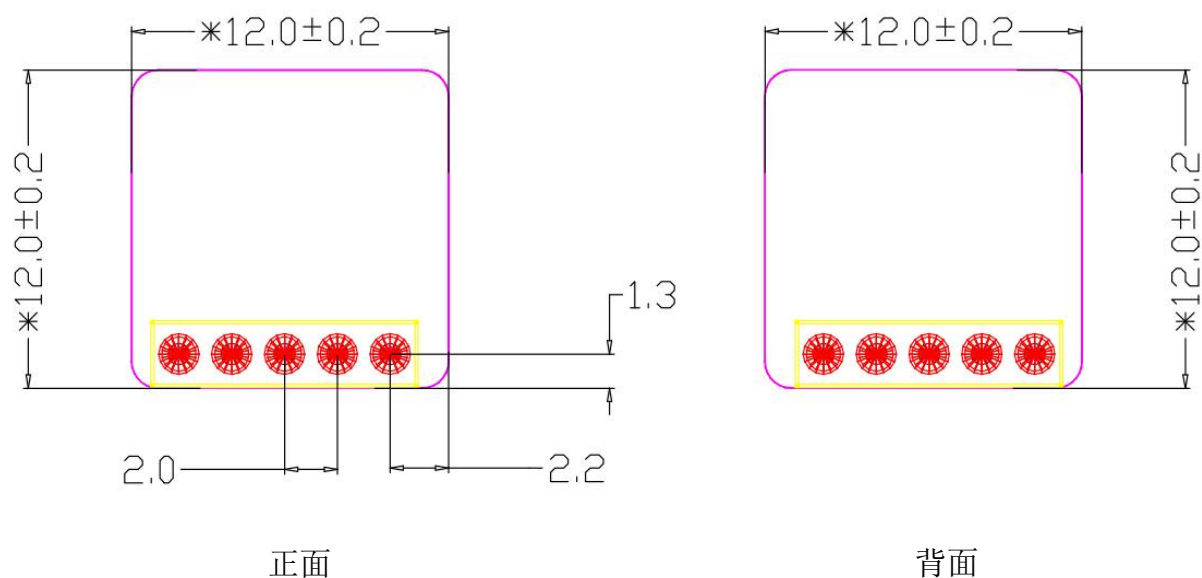
图 3 模组尺寸（单位：mm）
