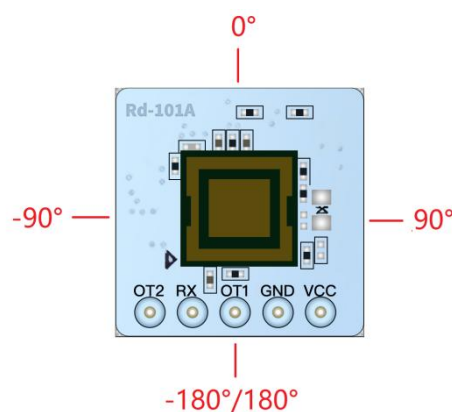
图 8 挂顶方向示意图
