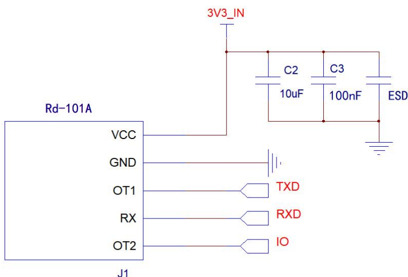
图 6 应用指导电路图
