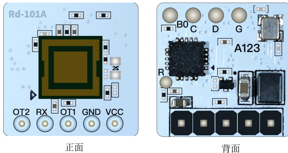
图 4 管脚示意图
