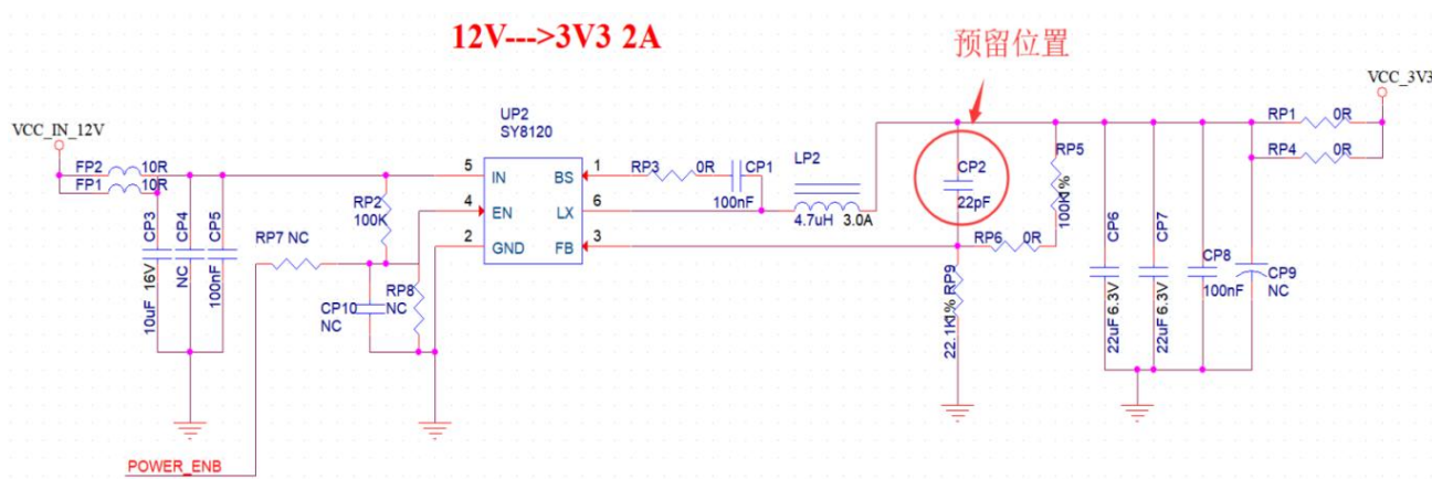
图 11 DC-DC 降压电路
