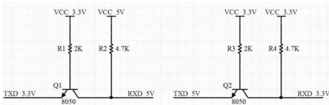
图 12 电平转换电路
