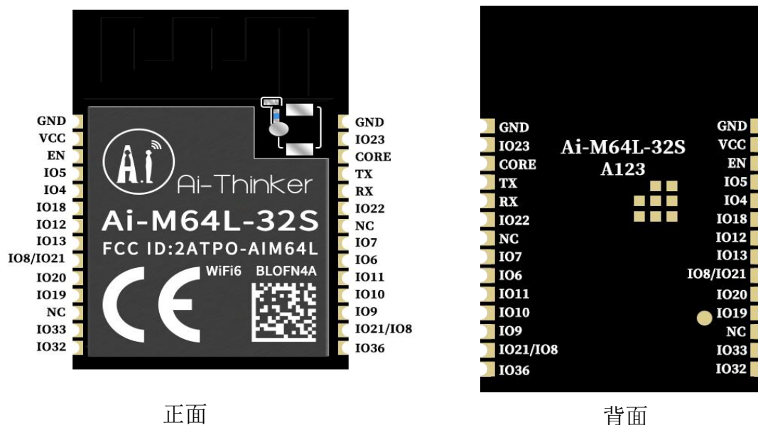
图 5 管脚示意图
