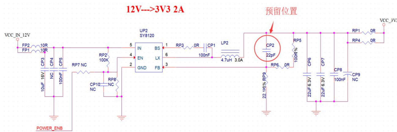
图 12 DC-DC 降压电路
