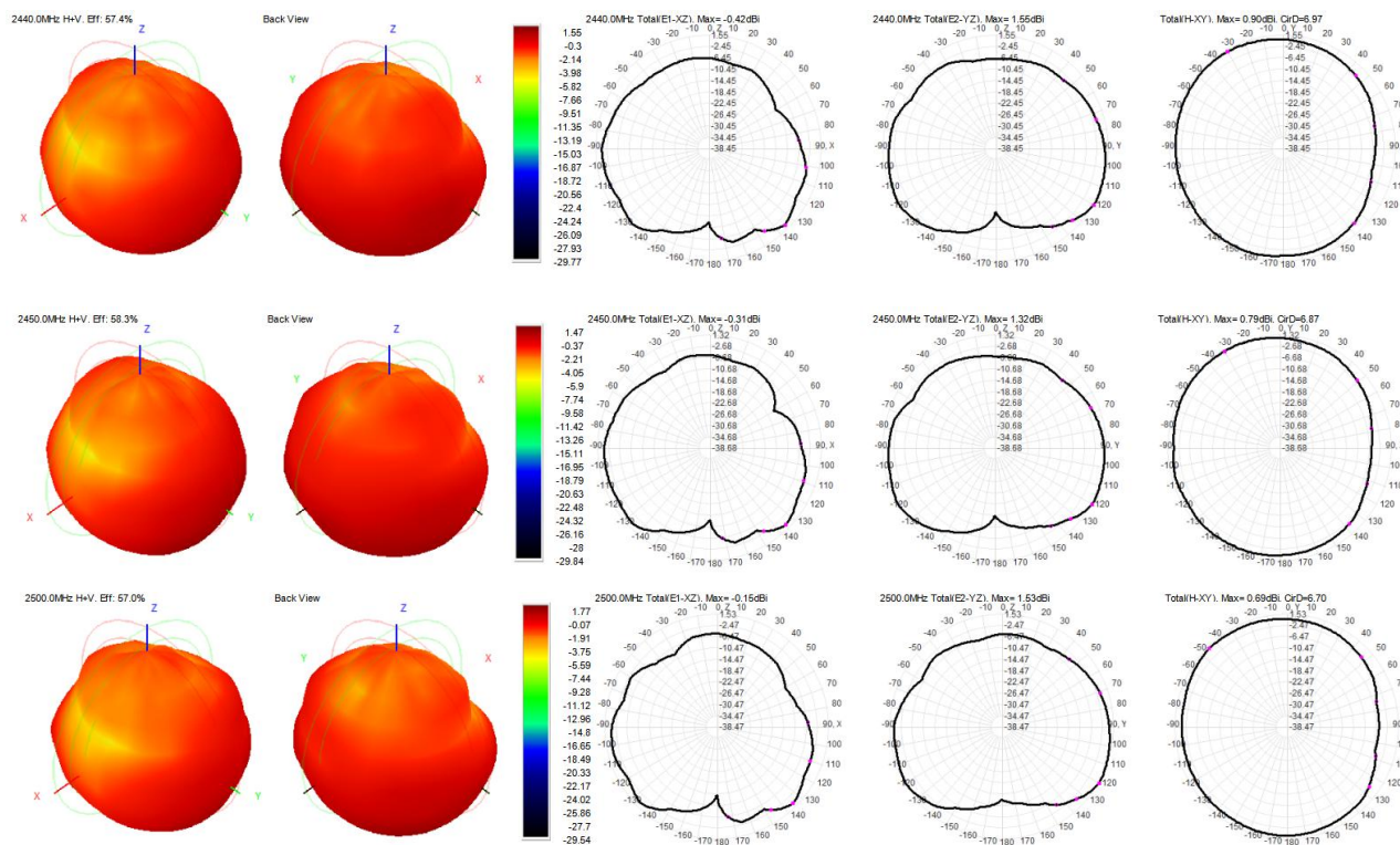
图 9 天线场型图
