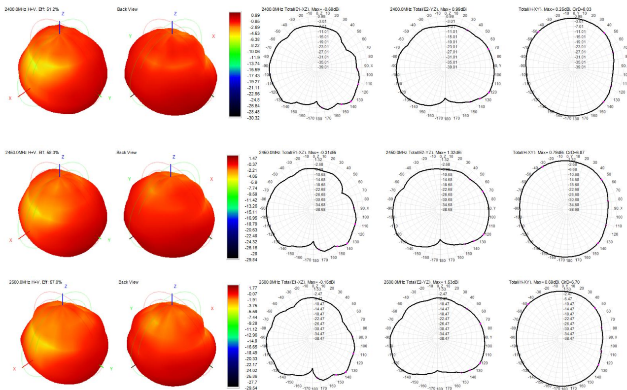
图 8 天线场型图
