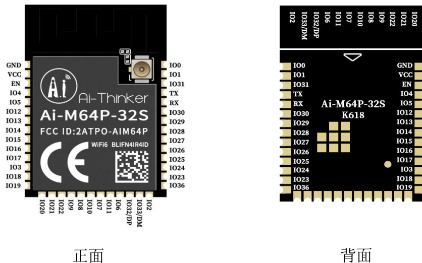
图 6 管脚示意图
