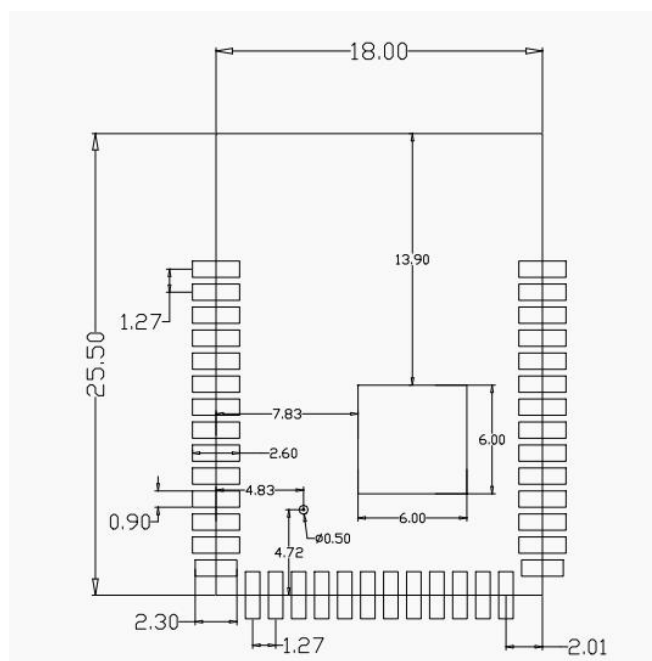
图 10 推荐 PCB 封装尺寸（单位：mm）
