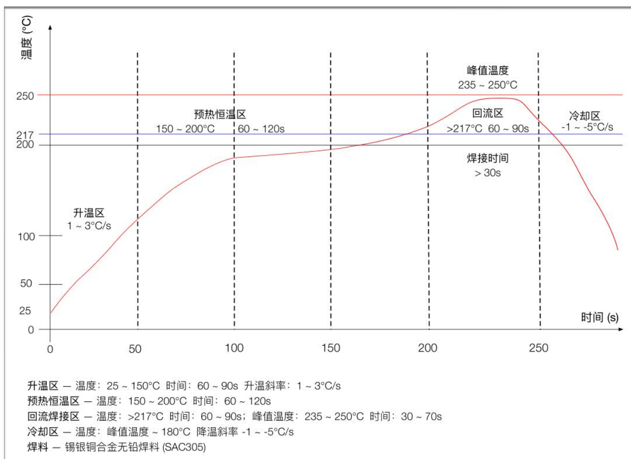
图 14 回流焊曲线
