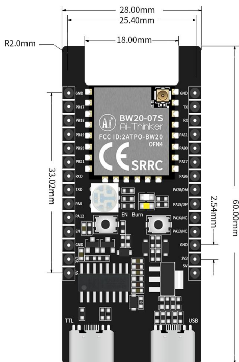
图 4 尺寸图
