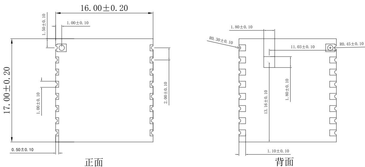
图 4 尺寸图（单位：mm）
