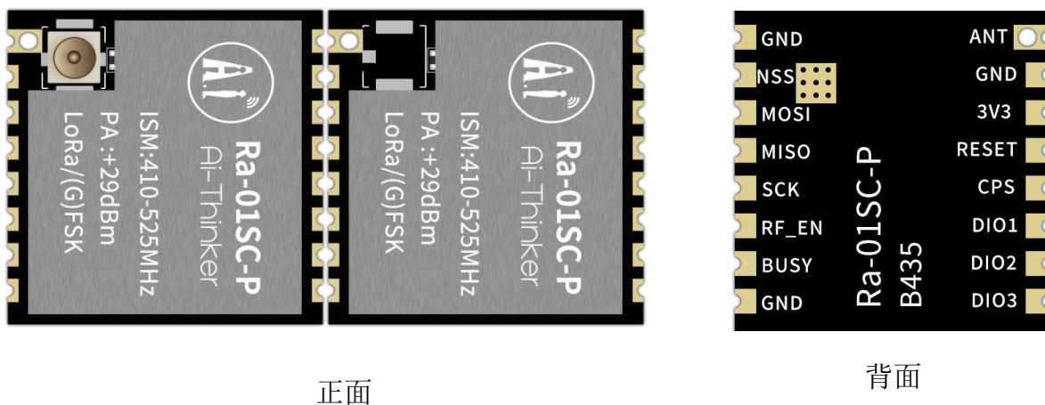
图 3 外观图（渲染图仅供参考，以实物为准）
