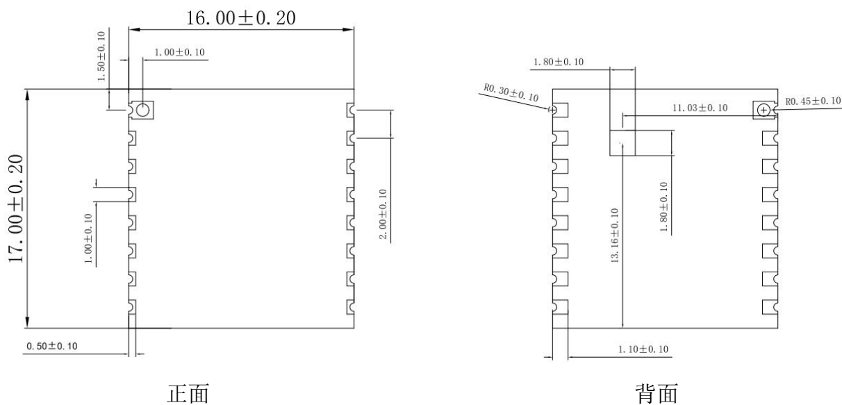
图 4 尺寸图（单位：mm）
