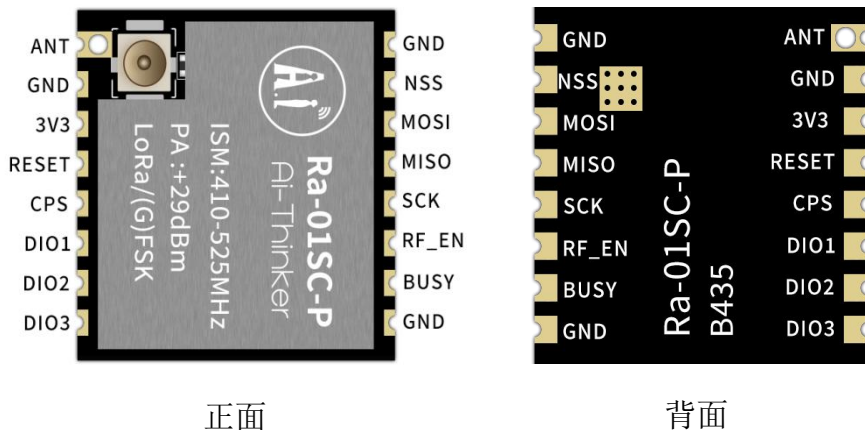
图 5 管脚示意图
