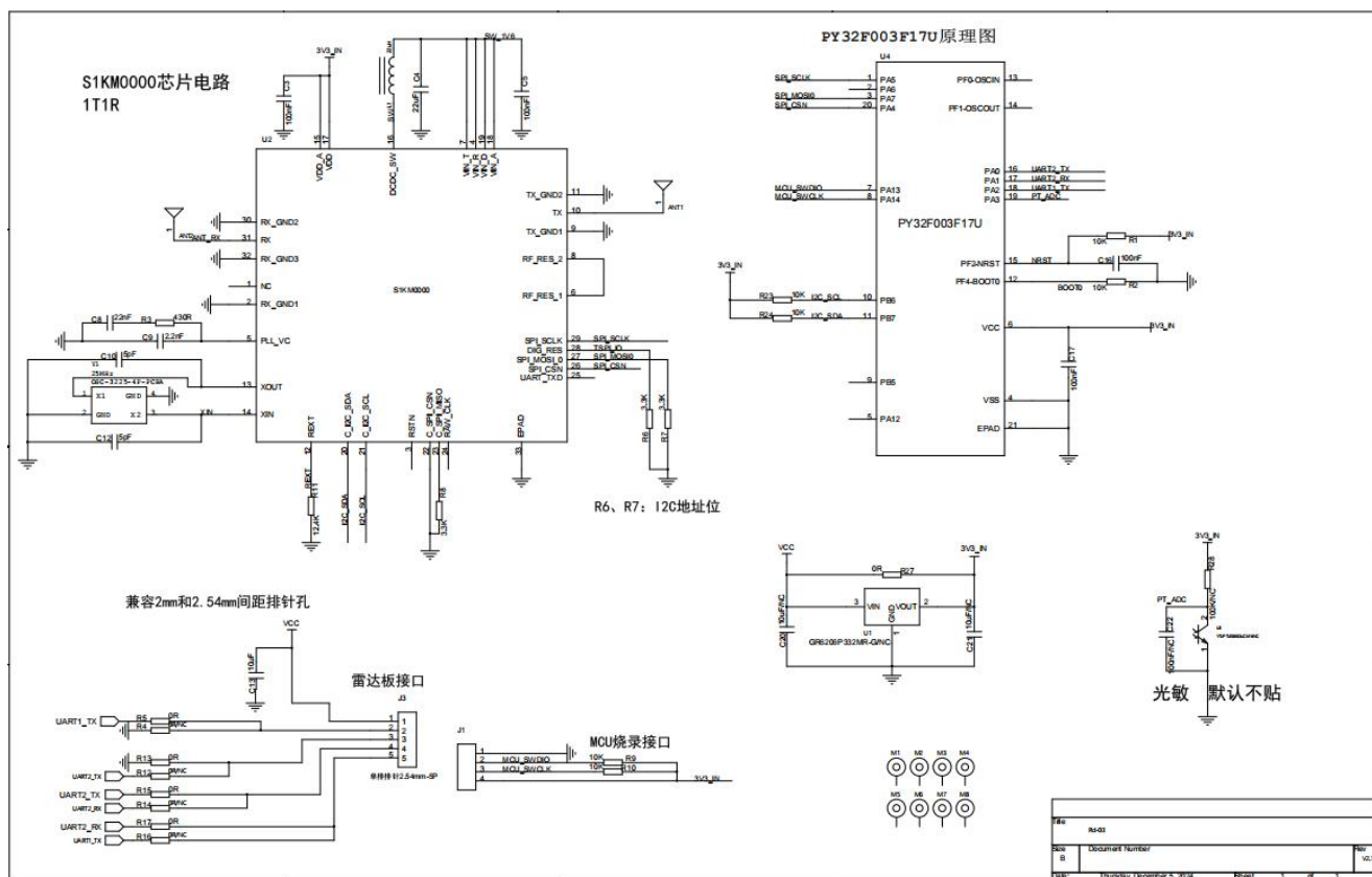
图 6 原理图
