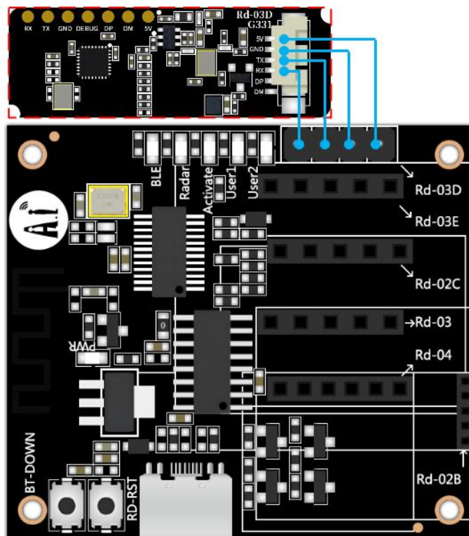
图 6 Rd-03D、Rd-03D_V2 接线示意图
