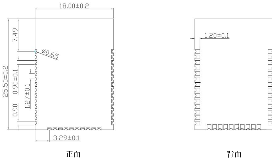
图 4 尺寸图
