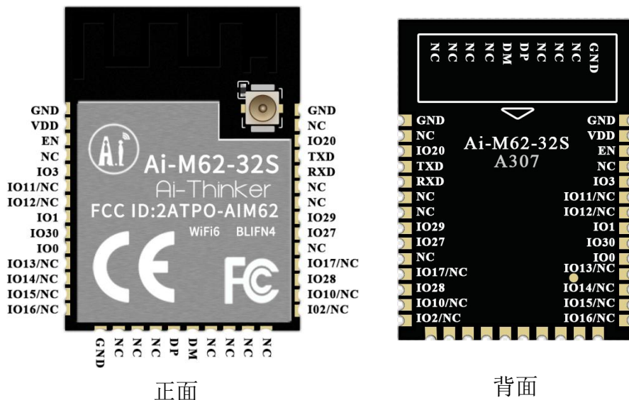
图 6 管脚示意图
