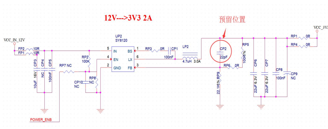
图 14 DC-DC 降压电路图
