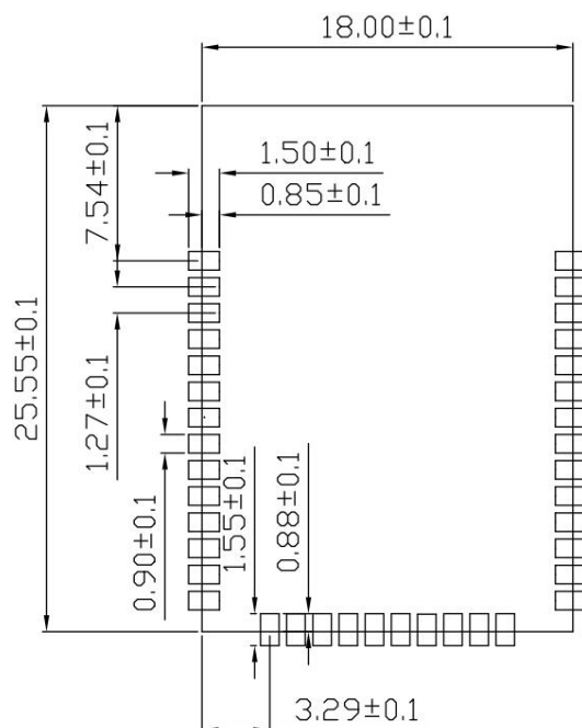
图 12 推荐 PCB 封装尺寸
