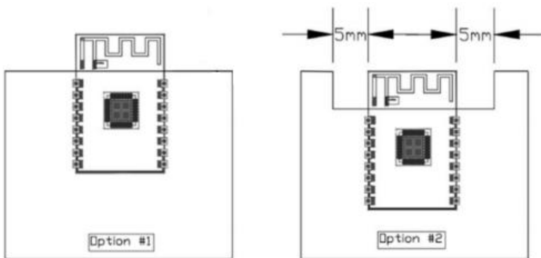
图 13 天线布局示意图
