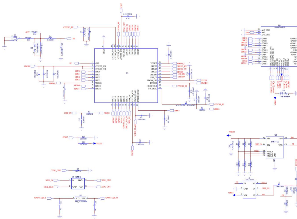
图 7 原理图
