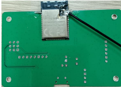
图 7 天线测试样机示意图
