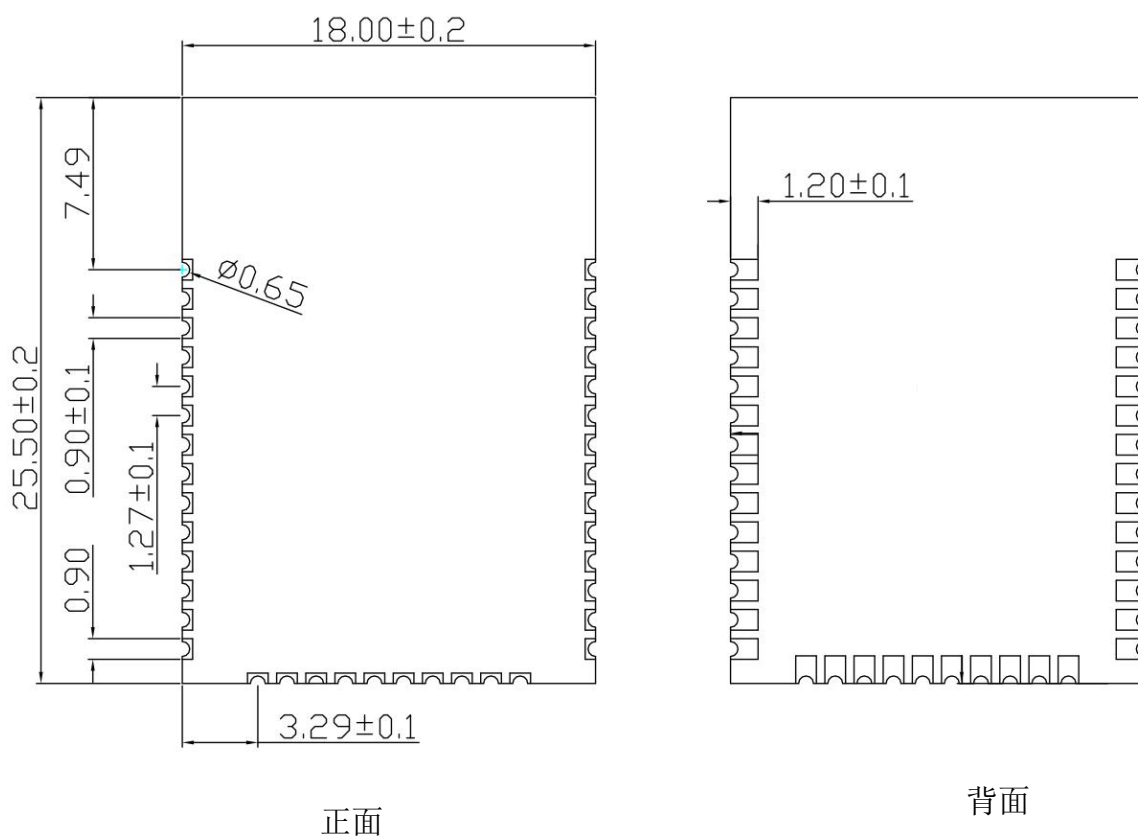
图 4 尺寸图
