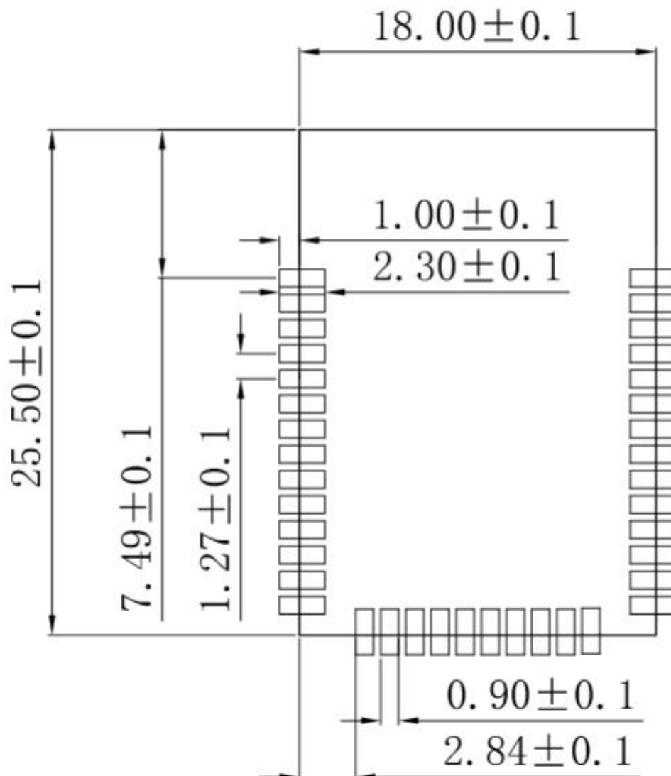
图 11 推荐 PCB 封装尺寸（顶视图）
