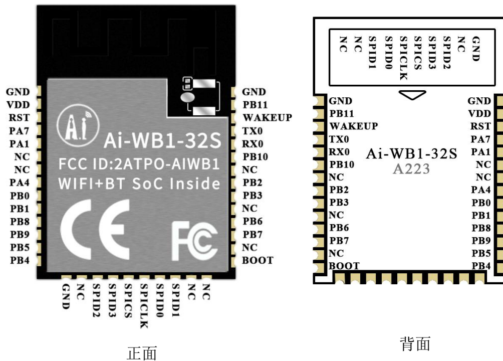
图 5 管脚示意图
