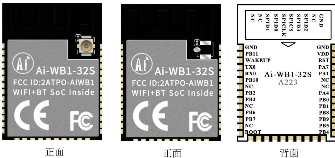
图 3 外观图（渲染图仅供参考，以实物为准）
