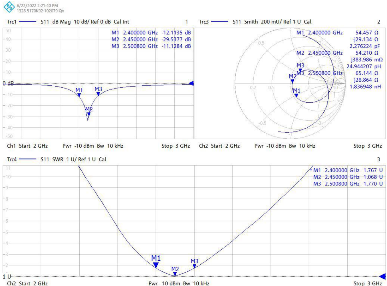
图 8 天线 S 参数
