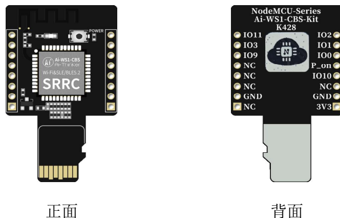
图 5 管脚示意图
