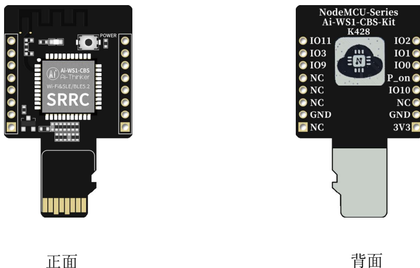
图 3 外观图（图片仅供参考，以实物为准）
