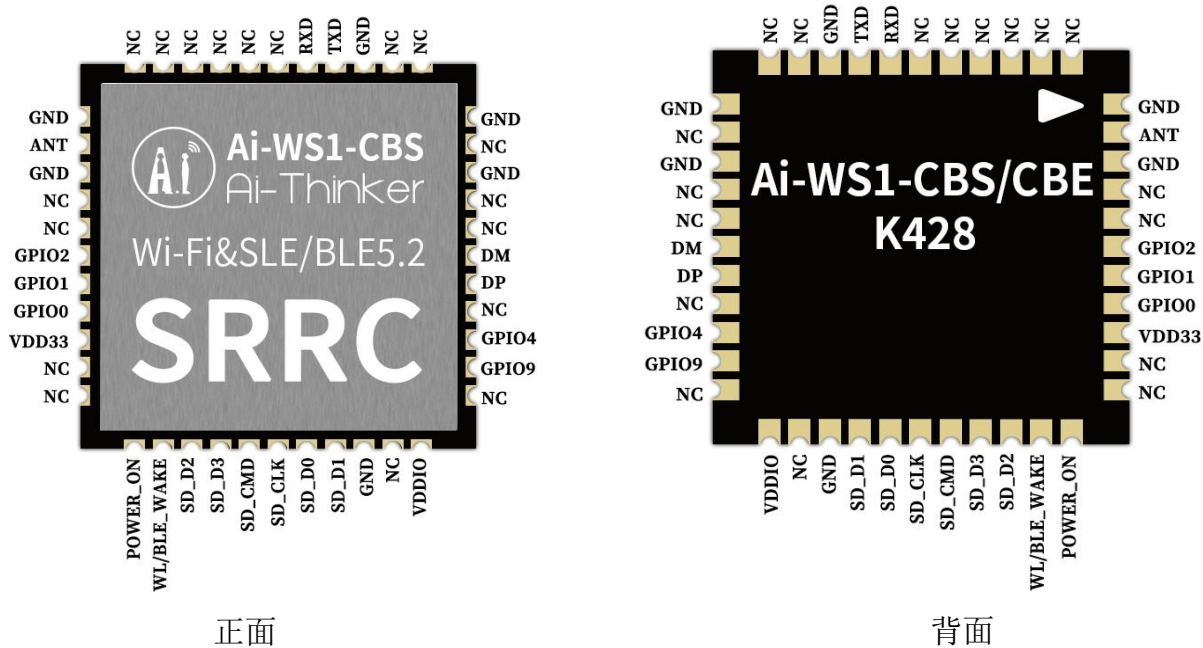
图 5 管脚示意图
