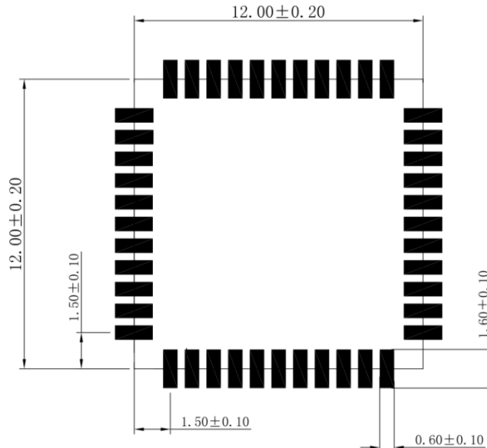
图 8 推荐 PCB 封装尺寸 (单位: mm)
