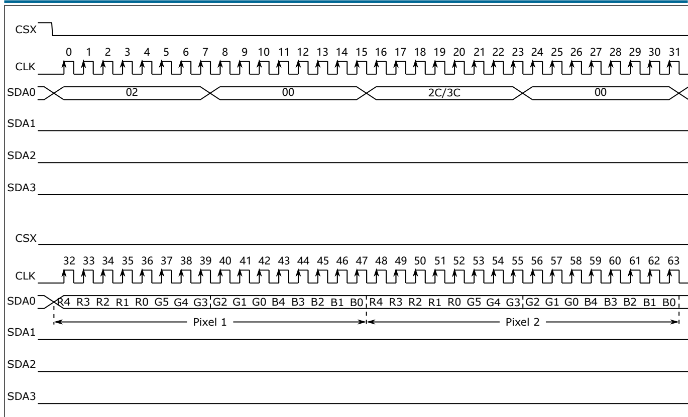
图 22.19: RGB565 输出
