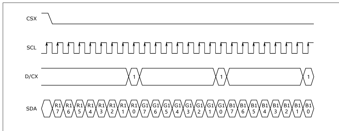
图 22.16: RGB888 输出
