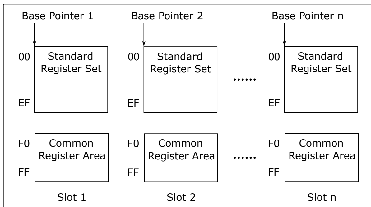
图 23.3: 多卡槽控制器的寄存器映射
