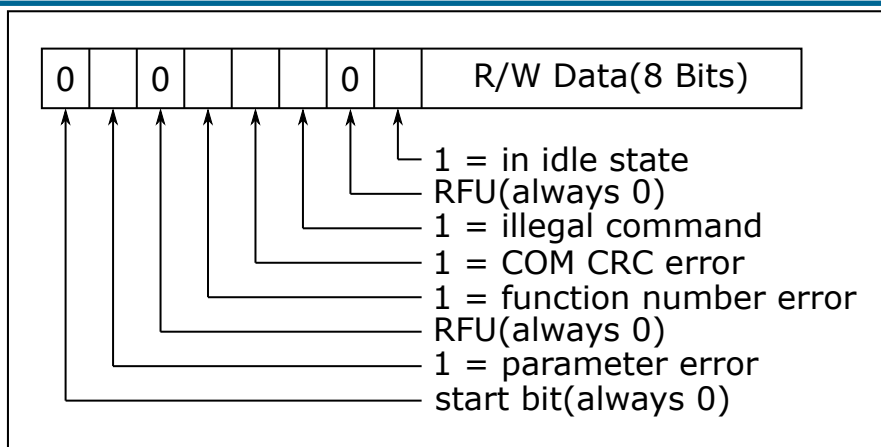
图 24.14: SPI 模式下的 IO_RW_DIRECT 响应
