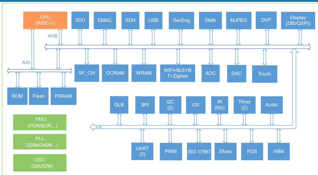
图 1.1: 系统框图
