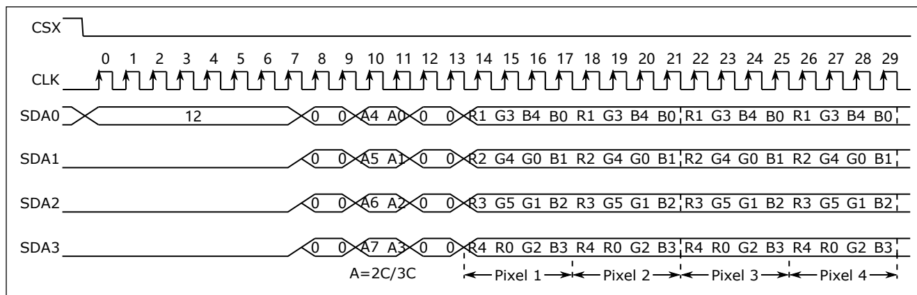
图 22.25: RGB565 输出
