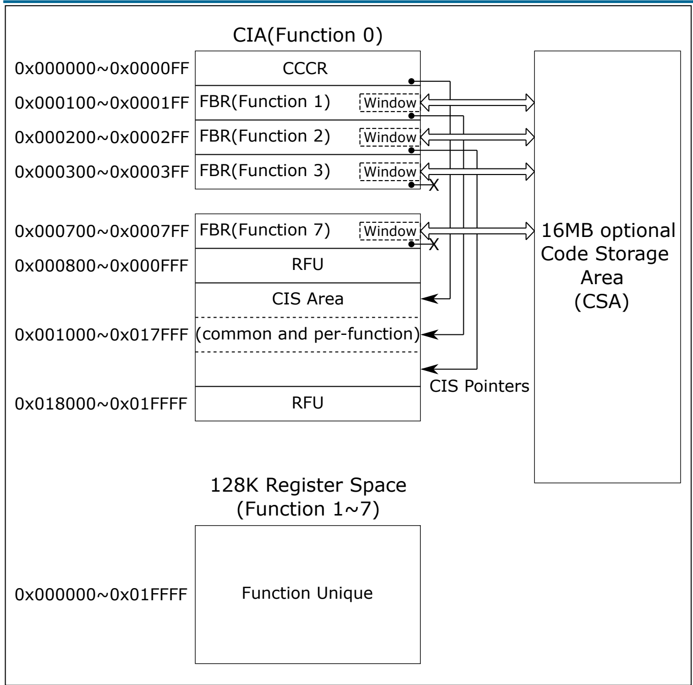
图 24.16: SDIO 内部映射
