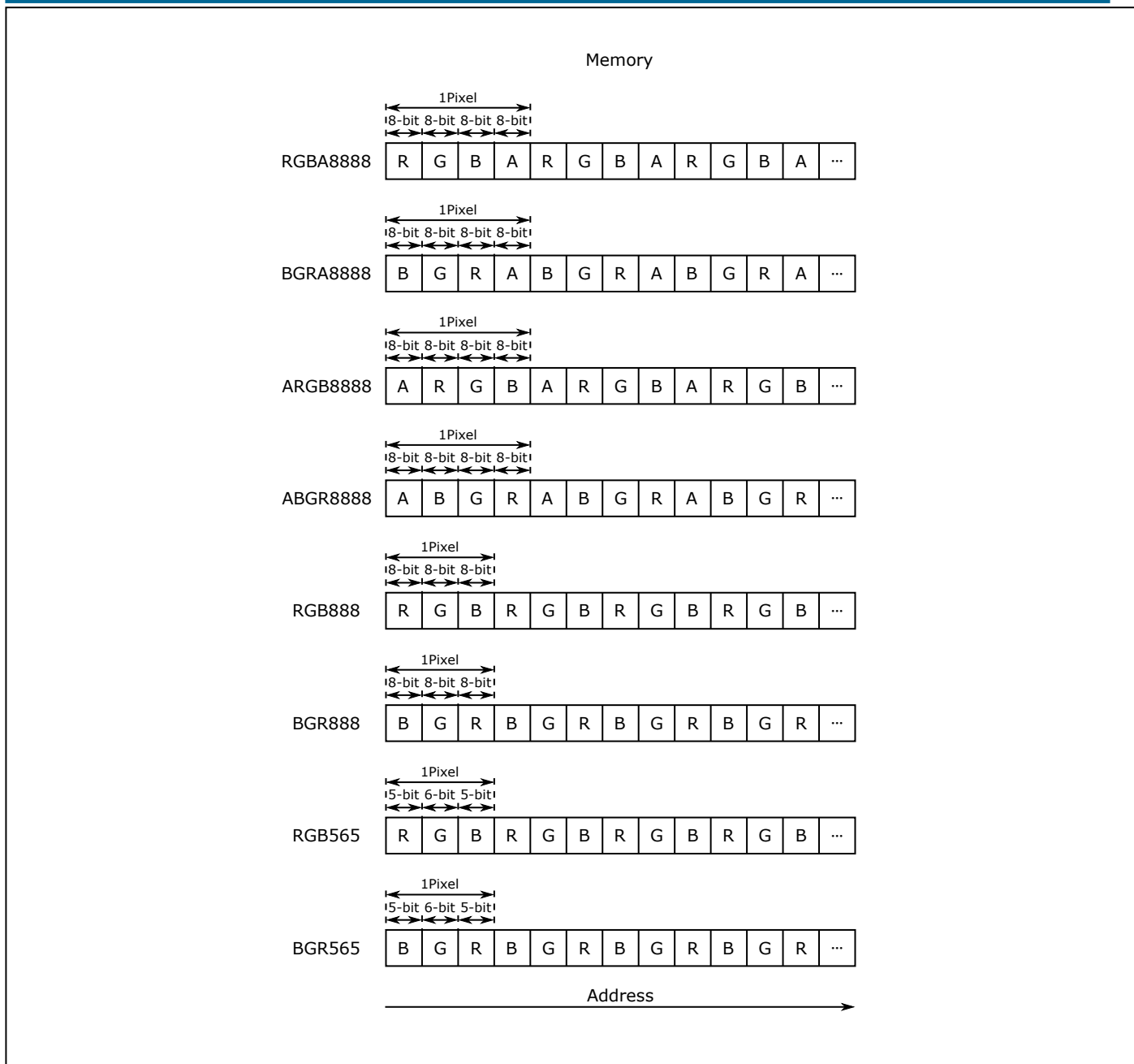
图 22.28: 输入像素 RGB 格式
