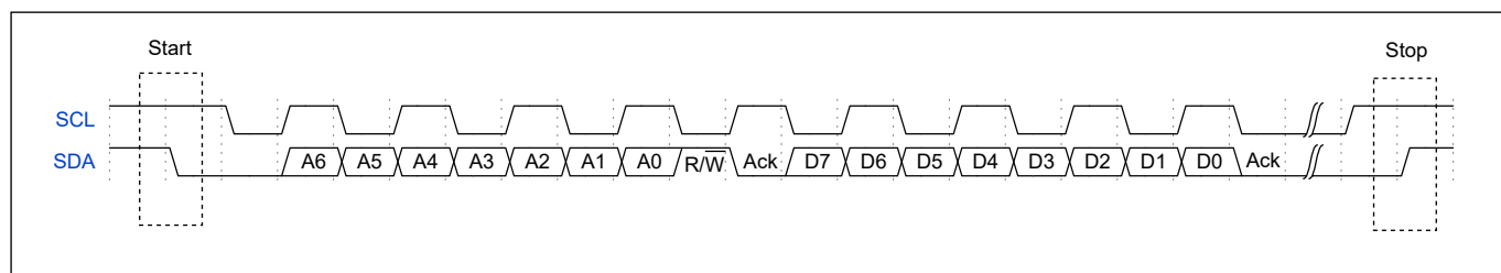
图 11.5: 主接收和从发送的时序
