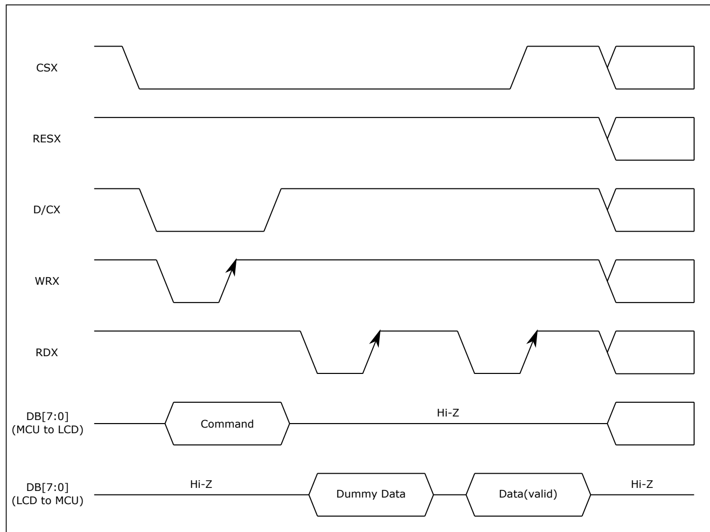
图 22.3: 读时序
