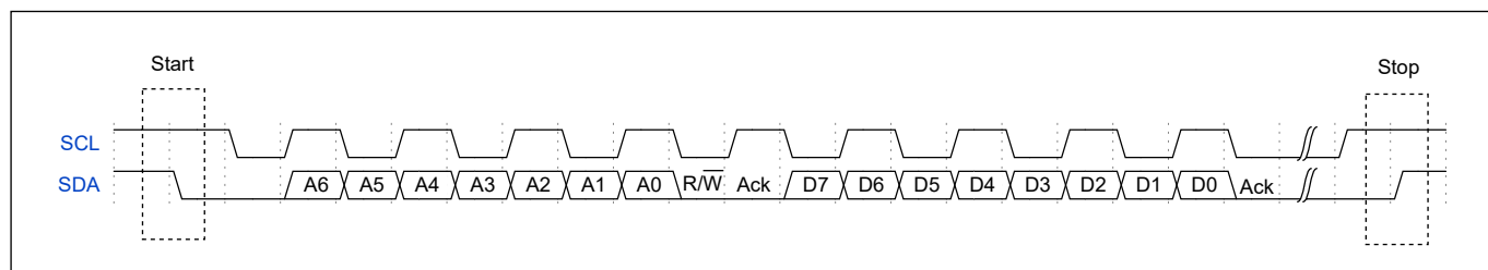
图 11.4: 主发送和从接收的时序
