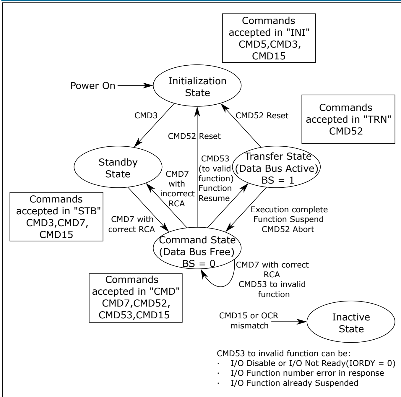
图 24.17: 总线状态机状态图
