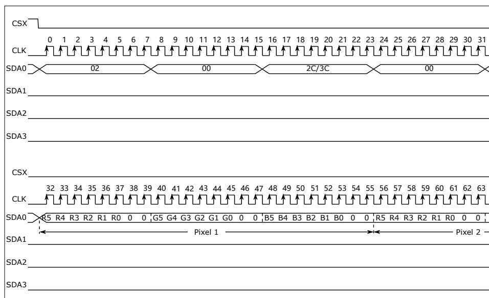
图 22.20: RGB666 输出
