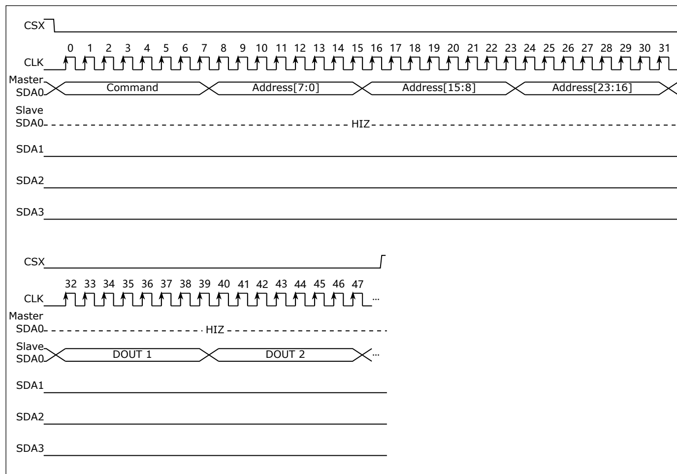
图 22.18: 读时序
