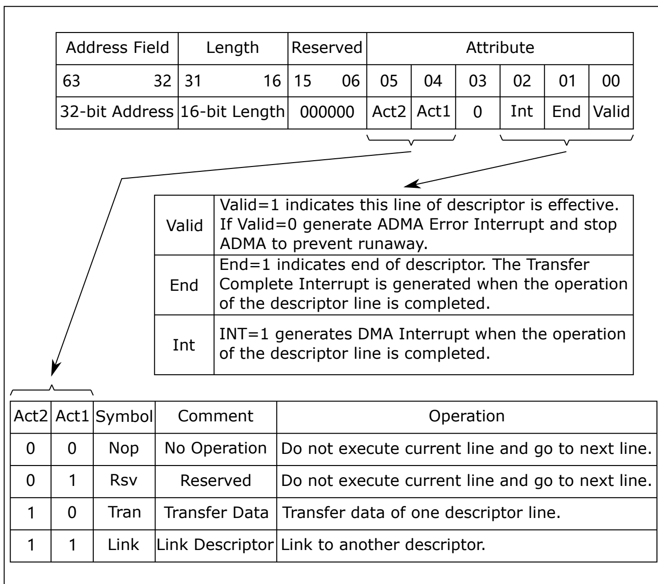
图 23.9: 32 位地址描述符表
