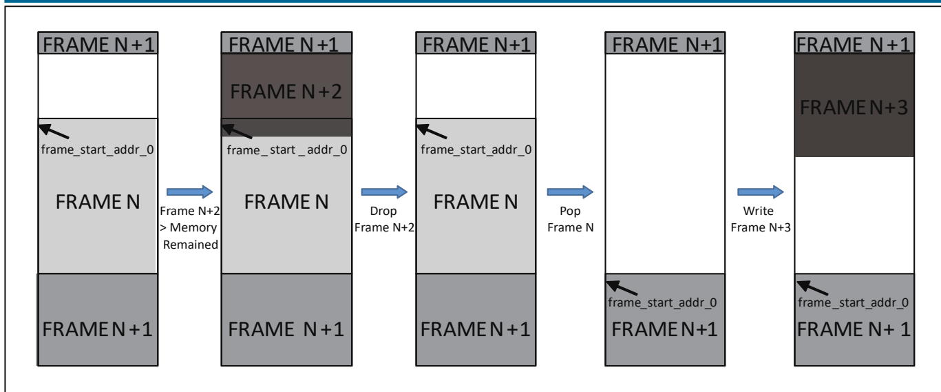
图 20.3: 内存
