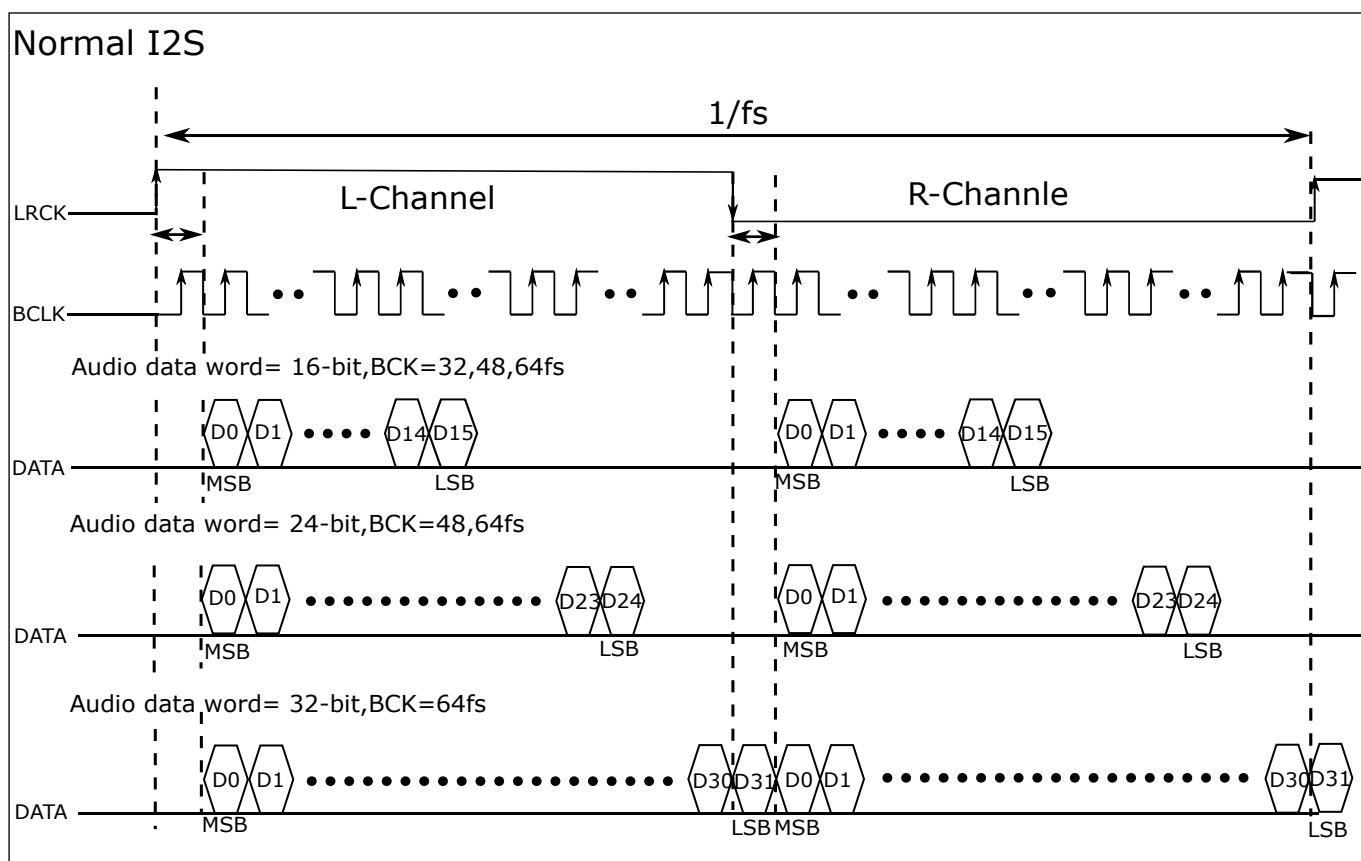
图 14.2: 标准 I2S 数据格式
