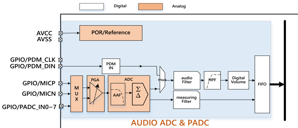
图 16.2: 模块框图
