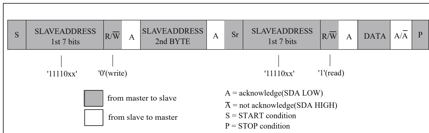
图 11.7: 主接收和从发送的数据格式 (10bit 从地址)
