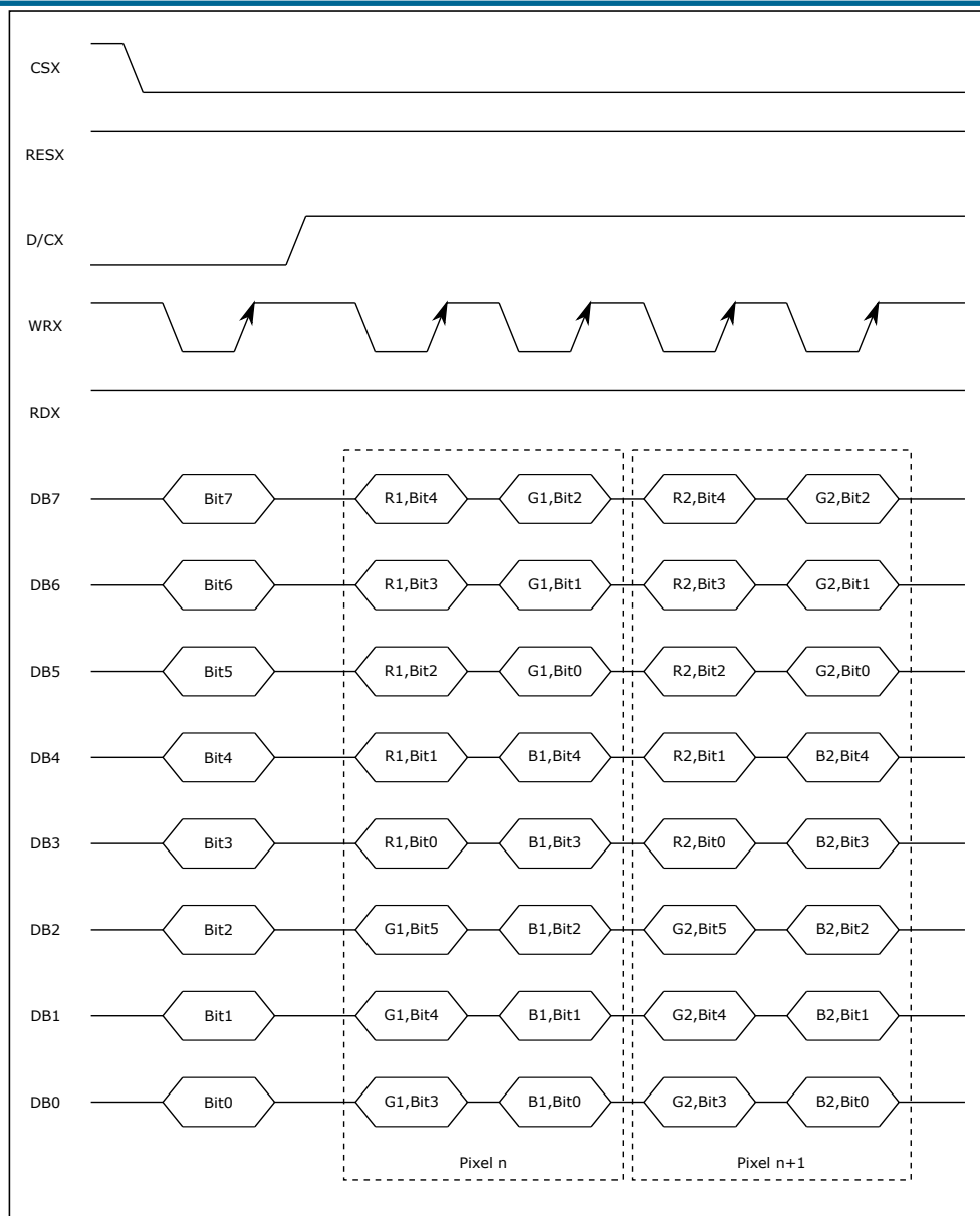
图 22.4: RGB565 输出
