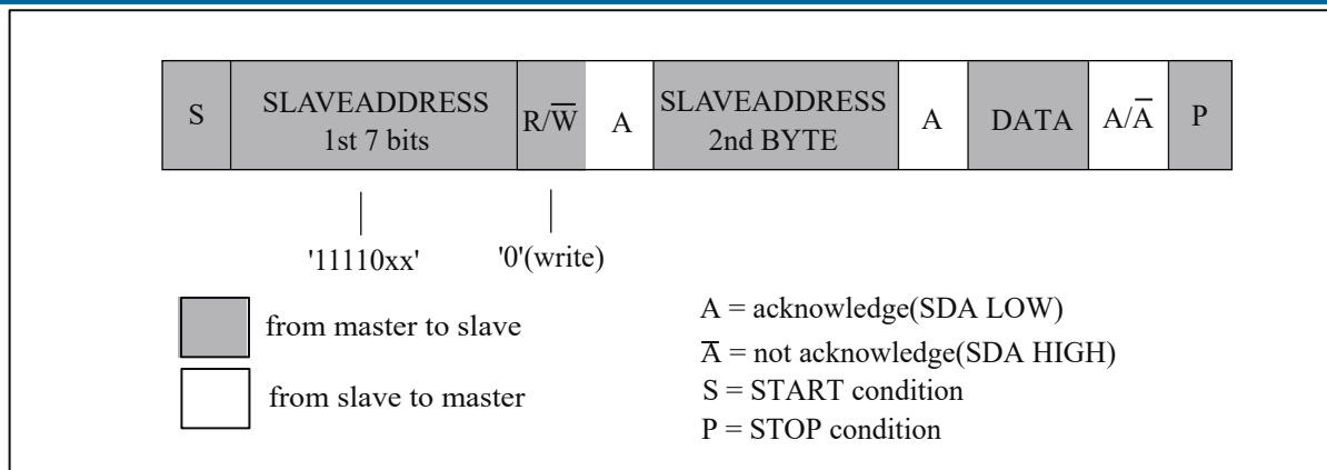
图 11.6: 主发送和从接收的数据格式 (10bit 从地址)
