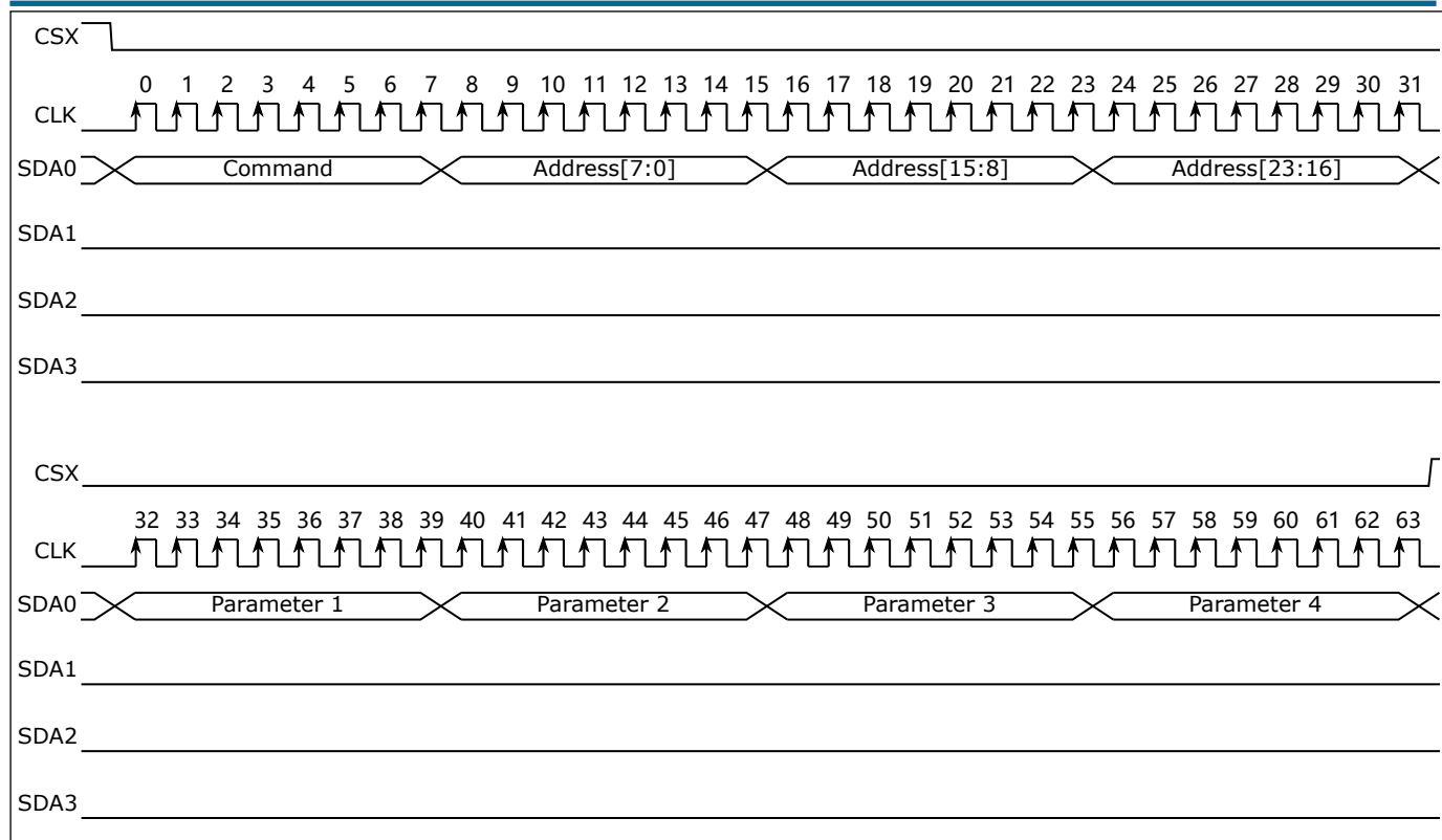
图 22.17: 写时序
