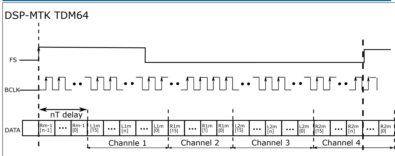
图 14.4: I2S TDM64 模式六通道录音
