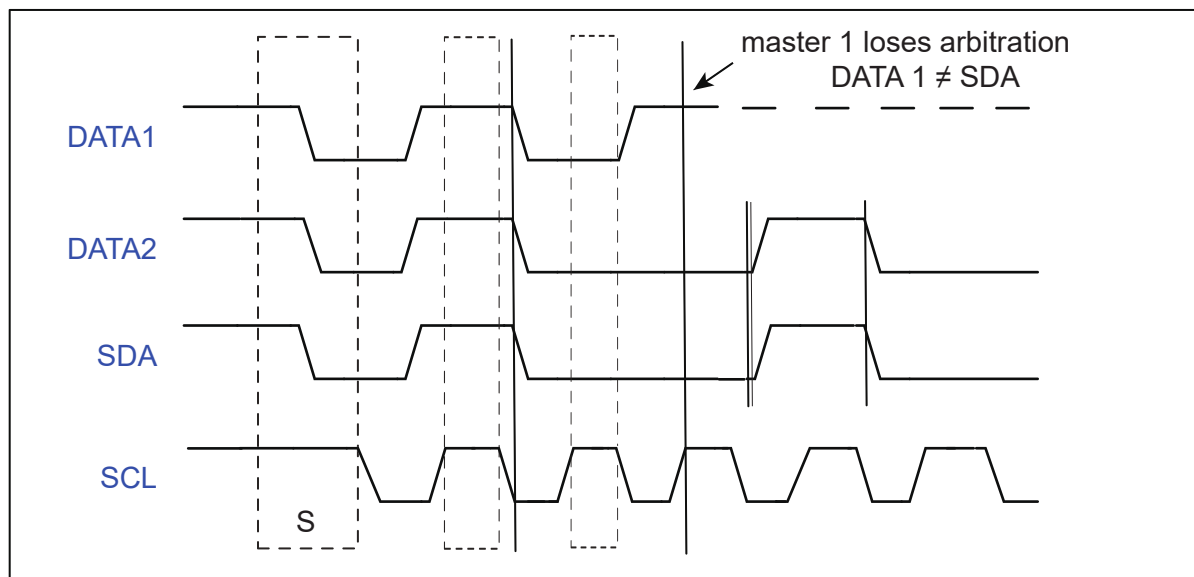
图 11.8: 同时传输数据波形示意图
