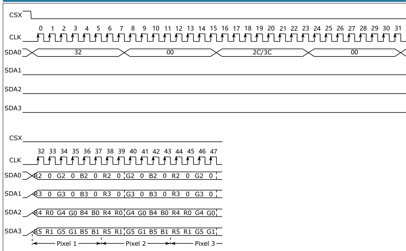
图 22.23: RGB666 输出
