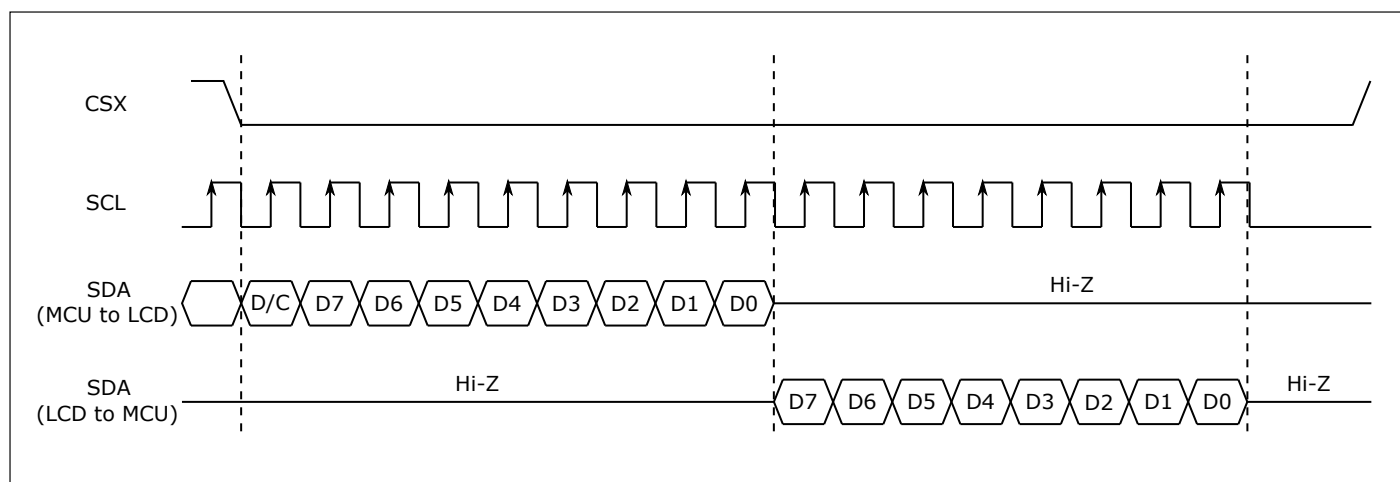
图 22.8: 读时序
