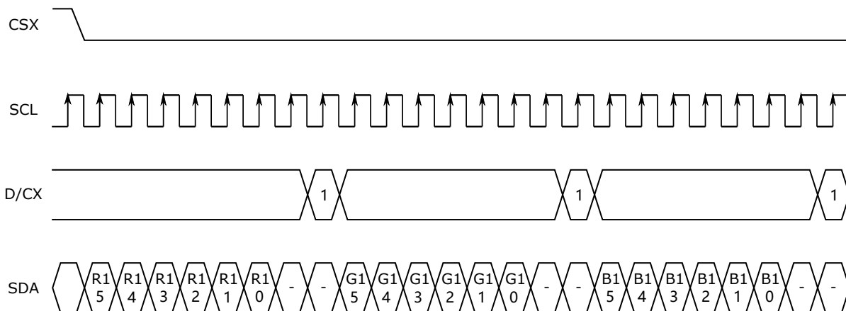
图 22.15: RGB666 输出
