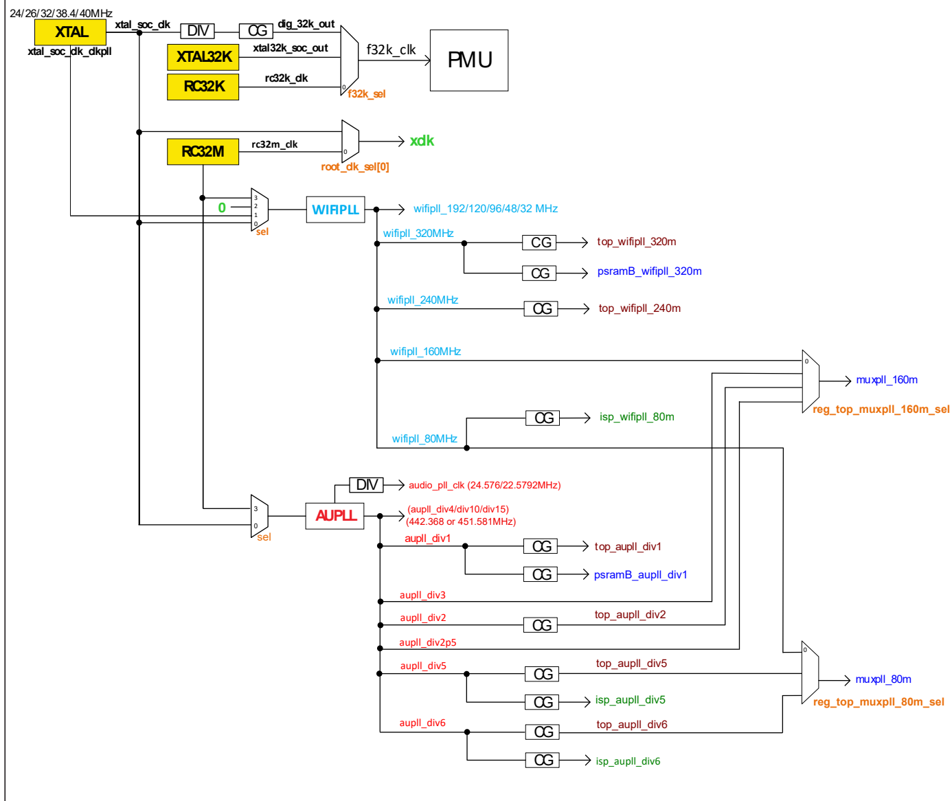
图 2.1: 系统时钟架构
