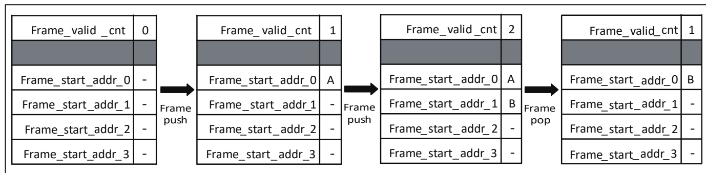
图 20.2: FIFO 框架
