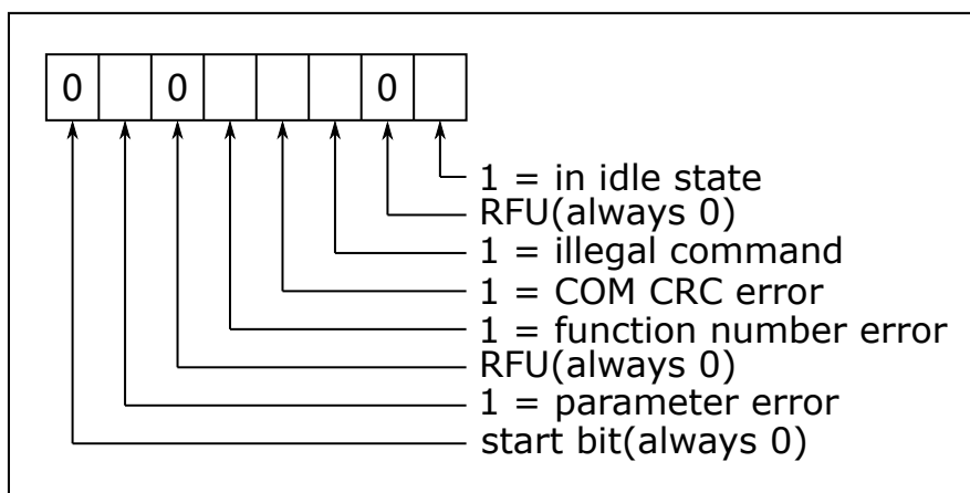
图 24.6: 改进的 R1 响应
