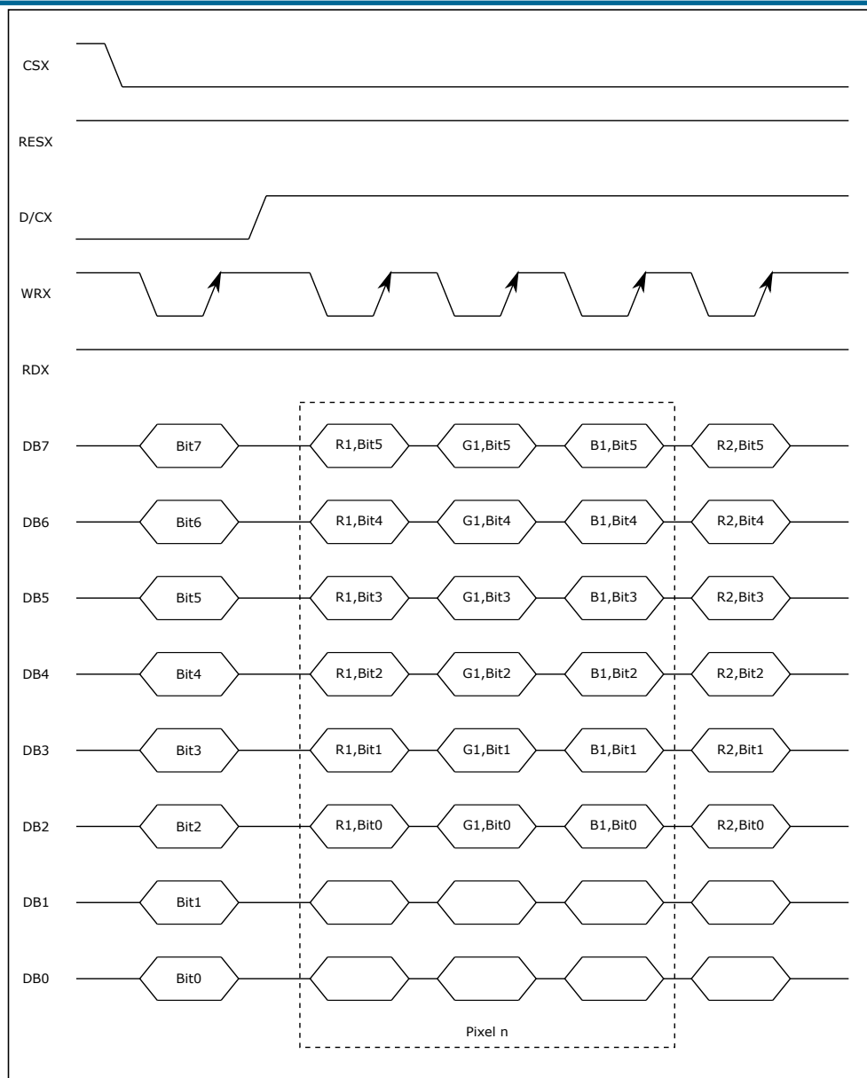
图 22.5: RGB666 输出
