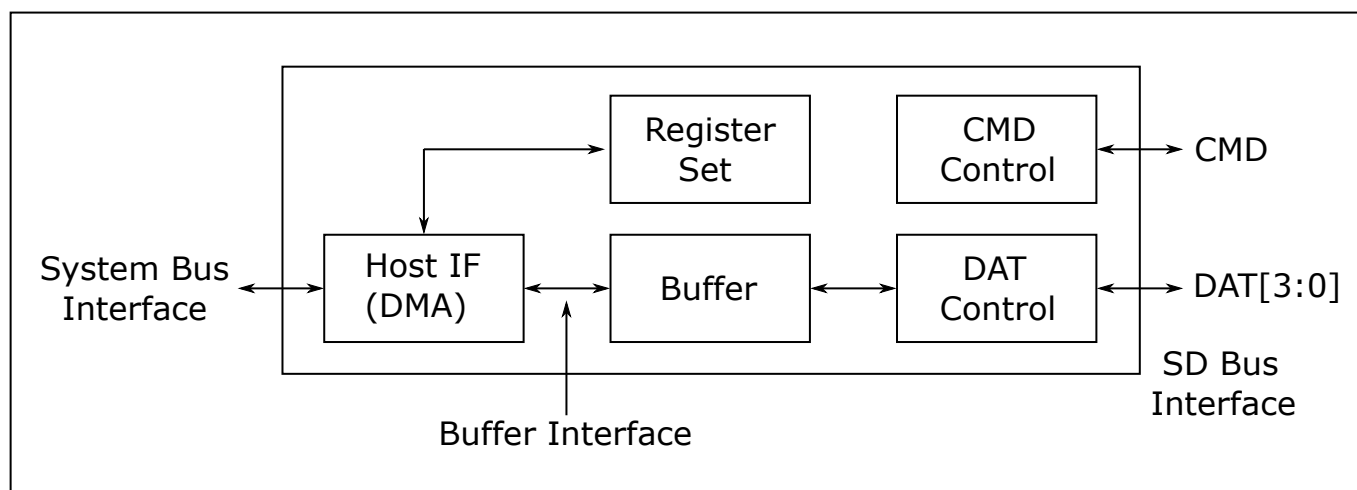
图 23.6: 主机控制器框图
