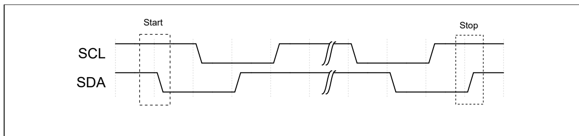
图 11.1: I2C 起始和停止条件
