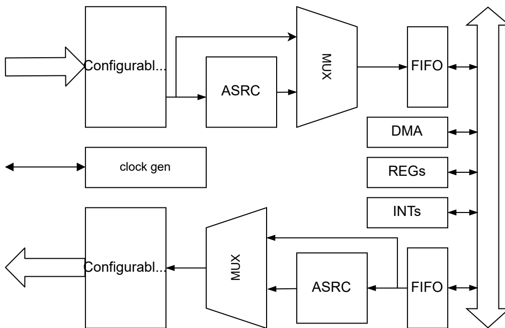
图 14.1: I2S 基本框图
