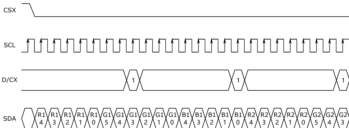
图 22.14: RGB565 输出
