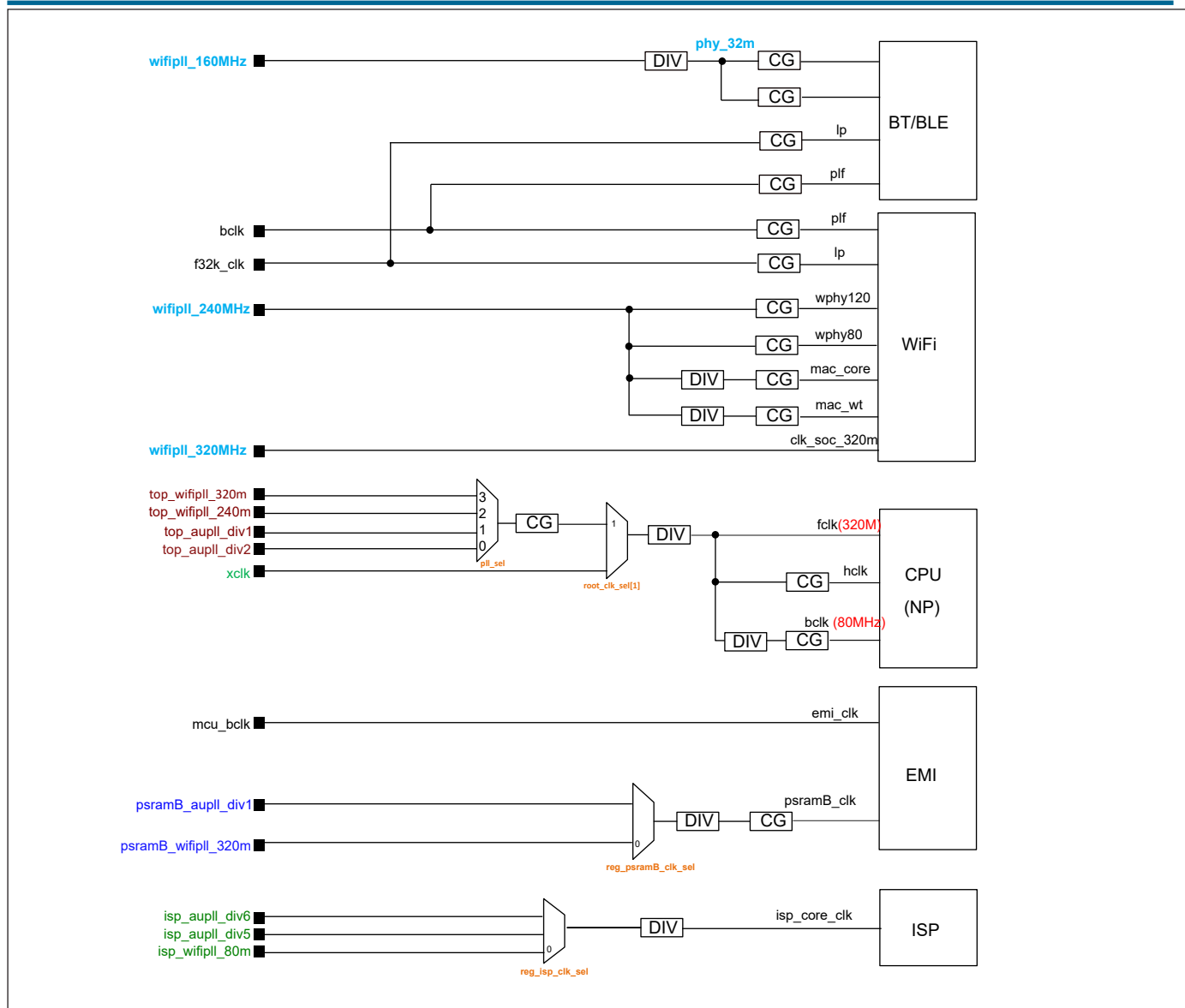
图 2.2: 模块时钟架构
