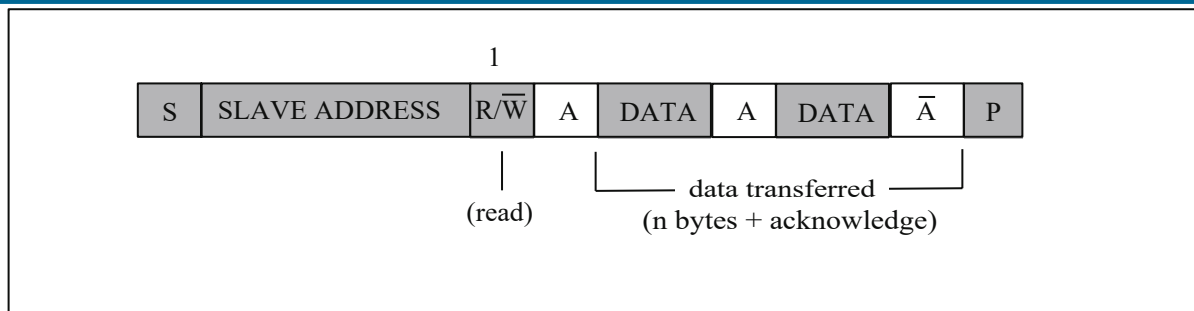
图 11.3: 主接收和从发送的数据格式
