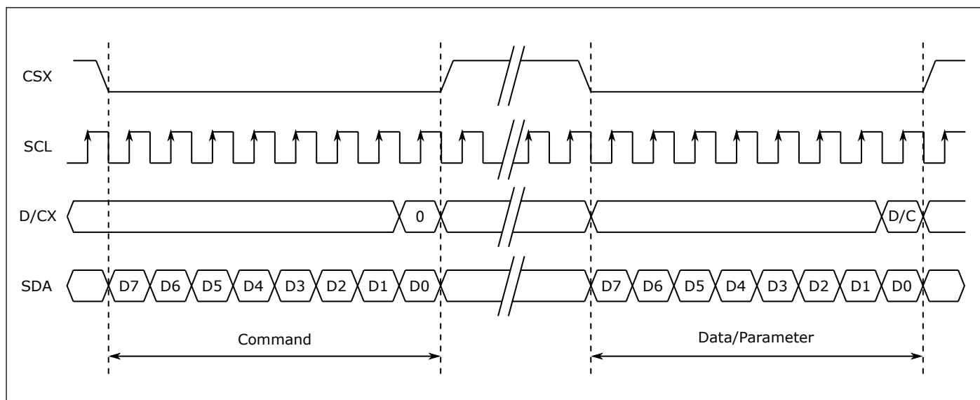
图 22.12: 写时序
