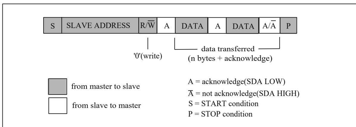
图 11.2: 主发送和从接收的数据格式
