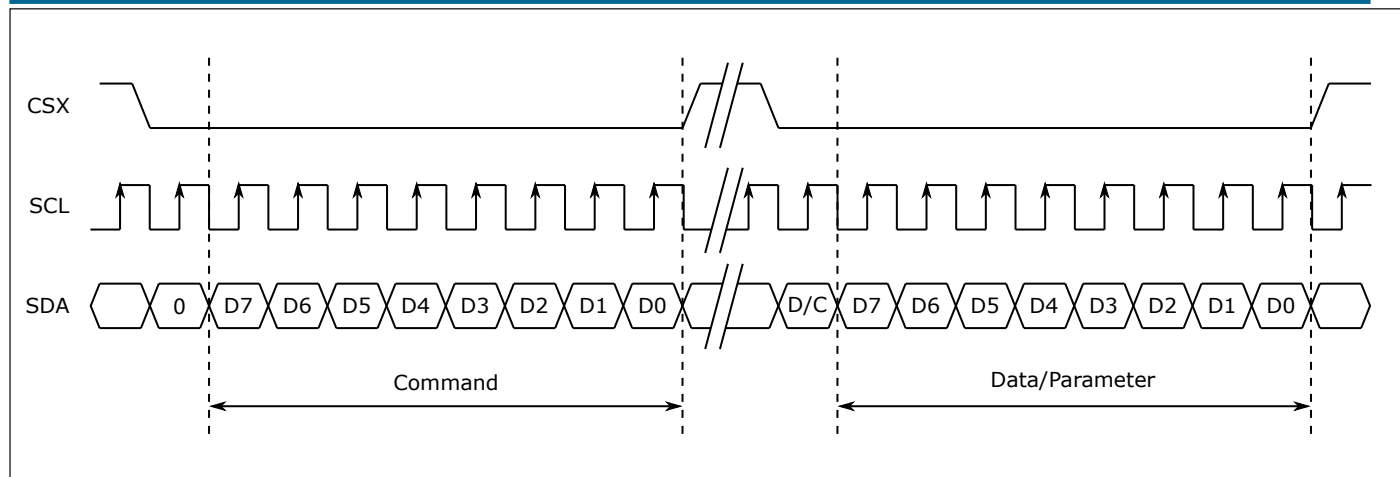
图 22.7: 写时序
