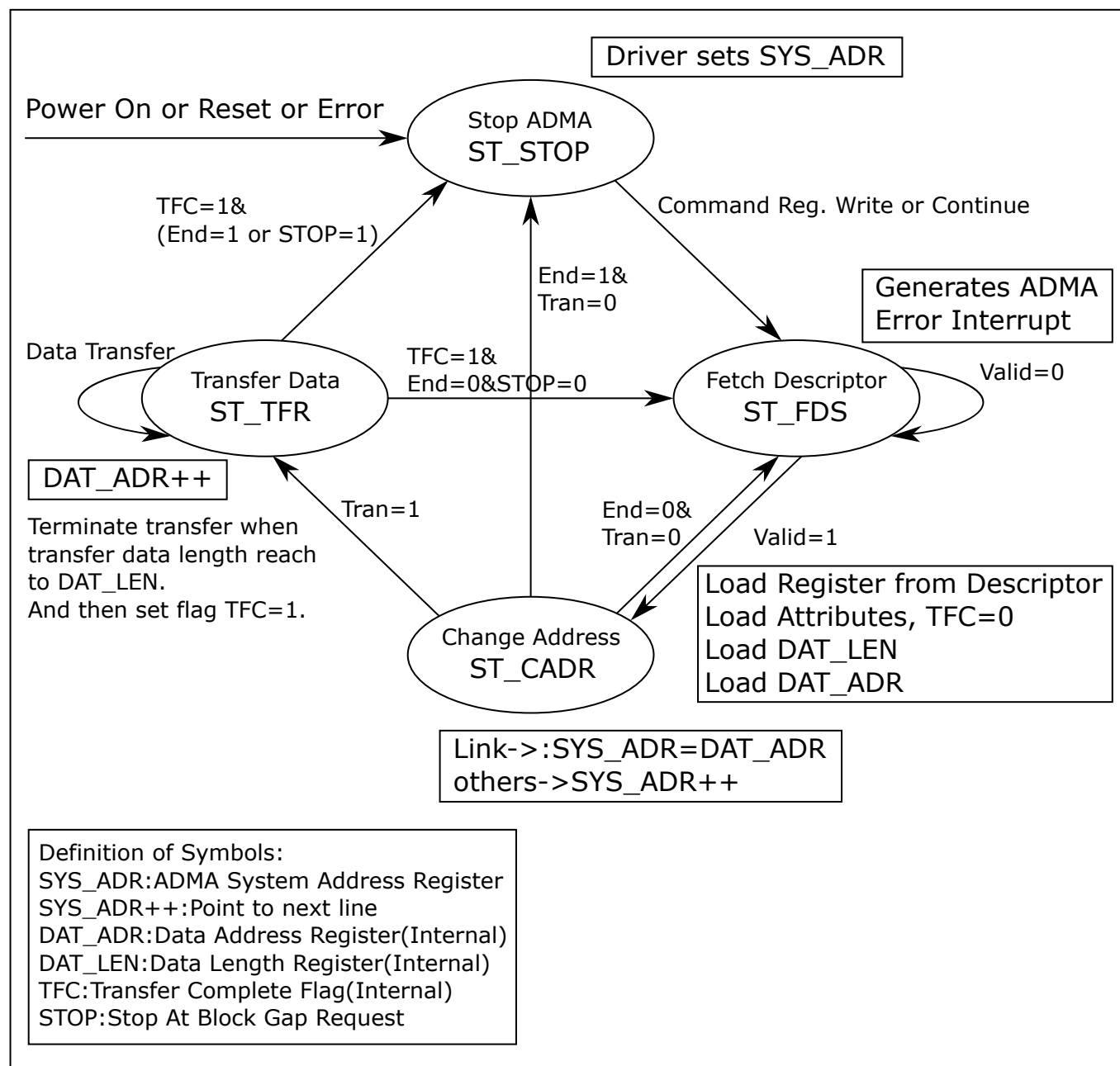
图 23.10: ADMA2 的状态图
