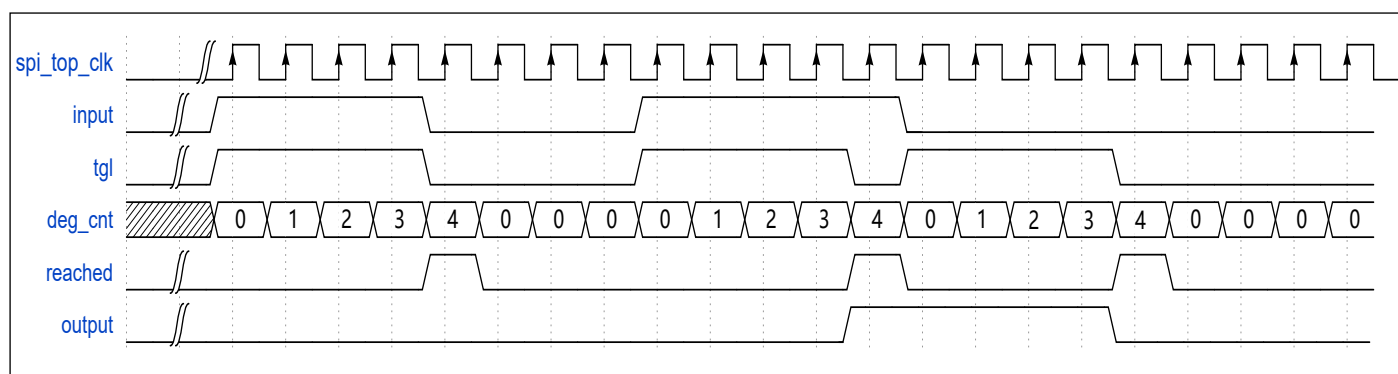
图 9.3: SPI 滤波波形图
