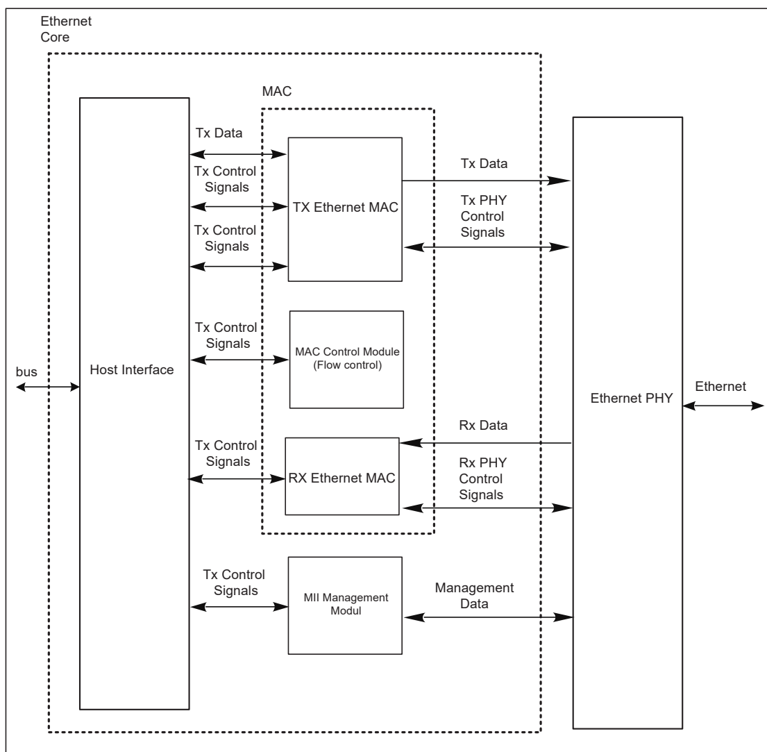
图 17.1: EMAC 框图
