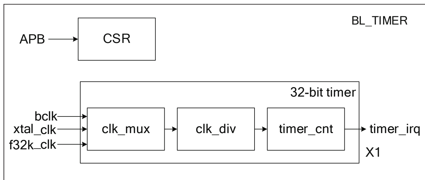
图 13.1: 定时器框图
