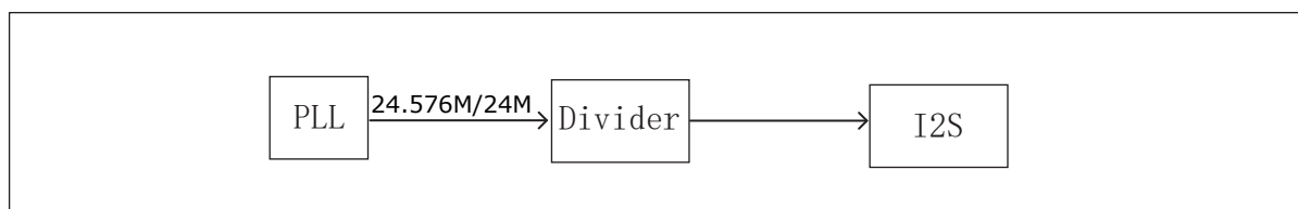
图 14.5: I2S 时钟
