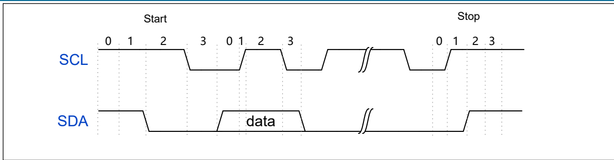
图 11.9: I2C 时钟设定
