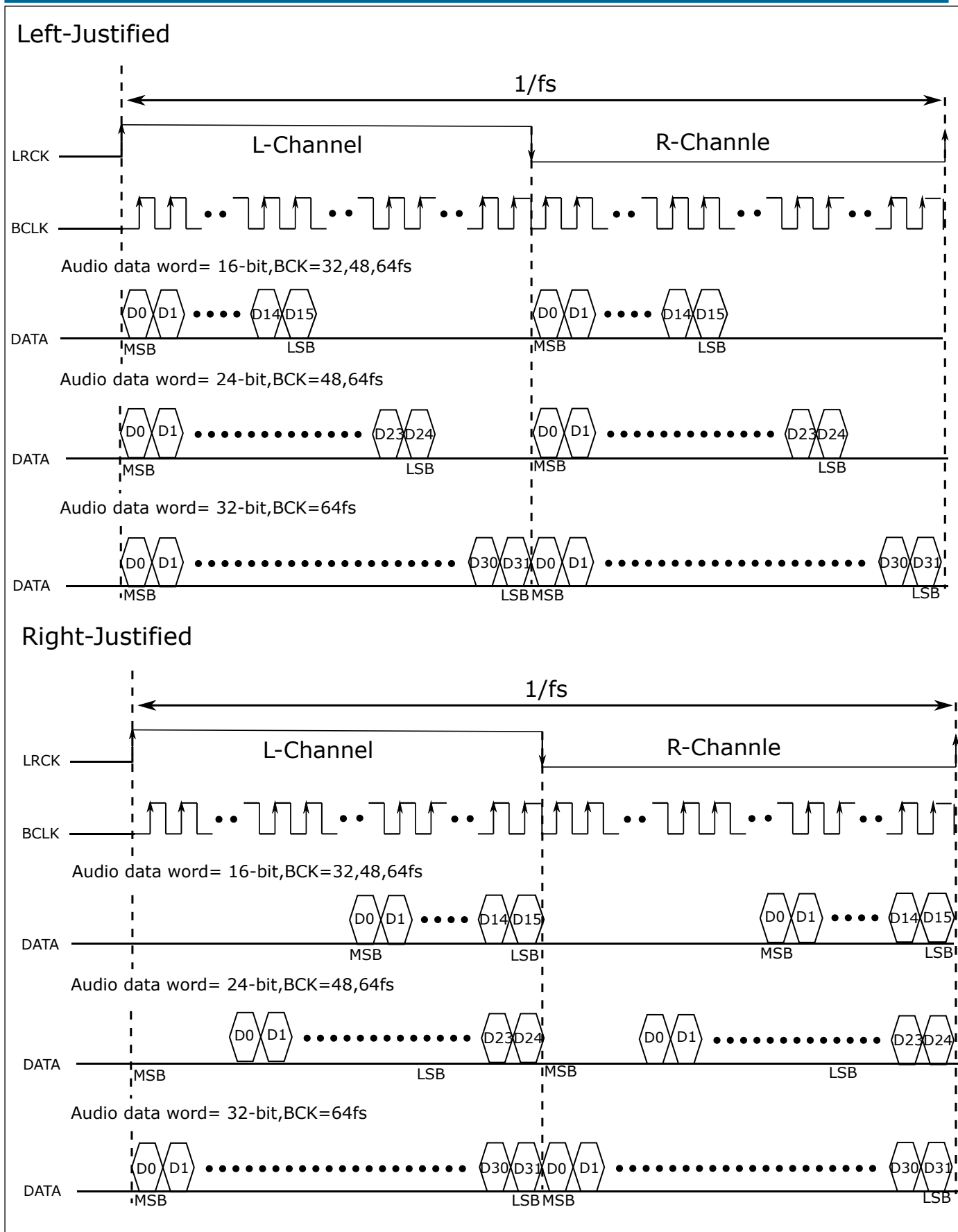
图 14.3: I2S 左对齐/右对齐数据格式
