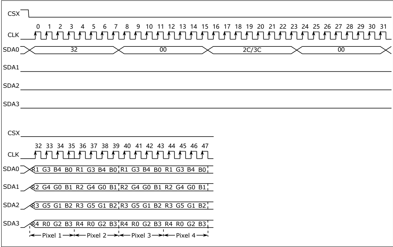
图 22.22: RGB565 输出
