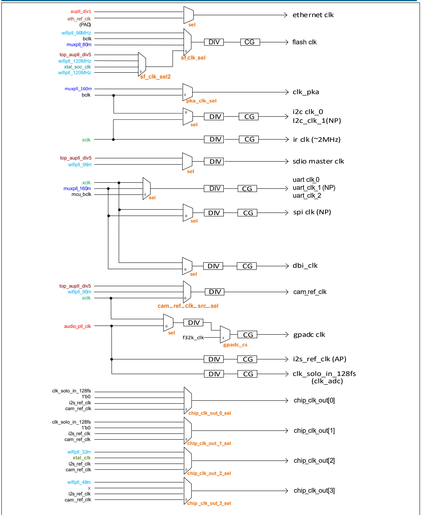
图 2.3: 外设时钟架构
