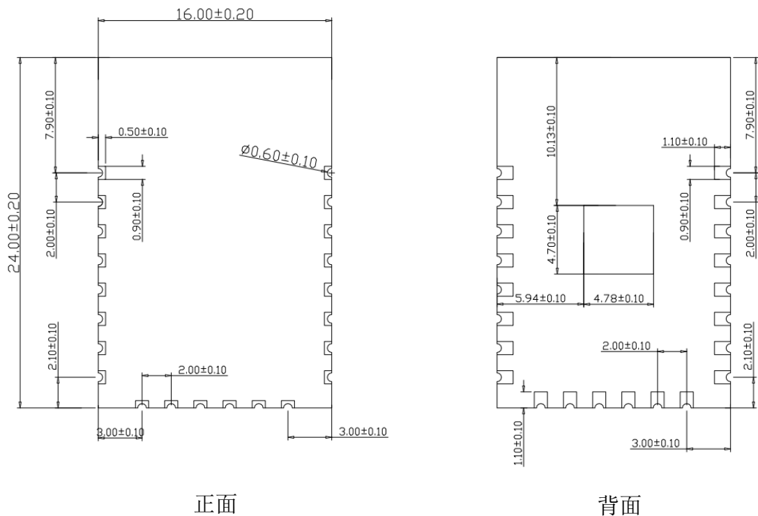
图 4 尺寸图
