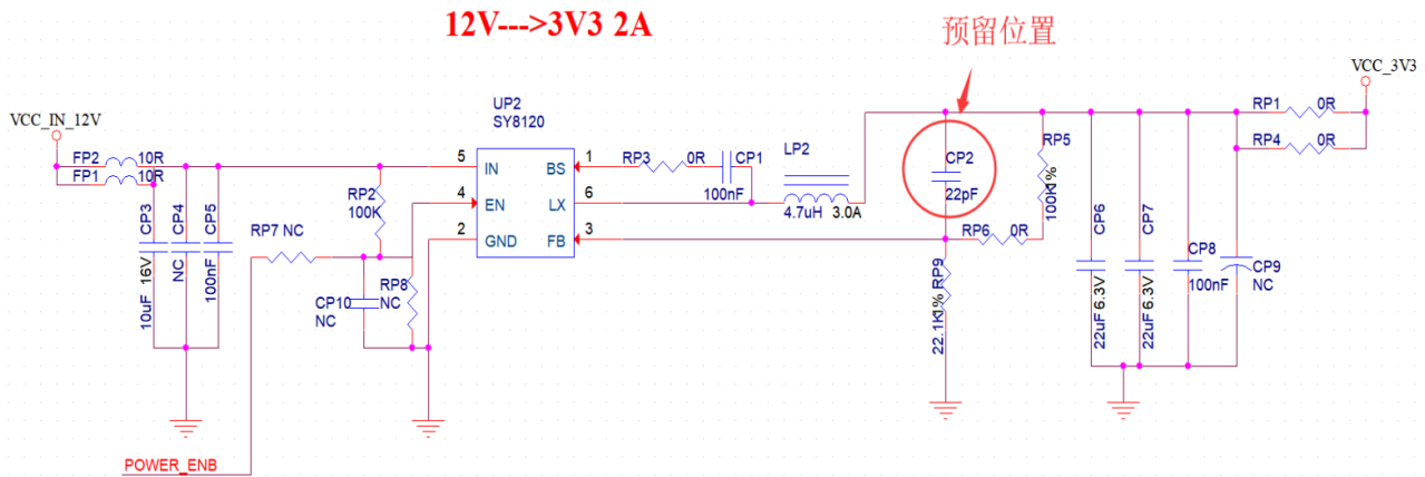
图 11 DC-DC 降压电路图
