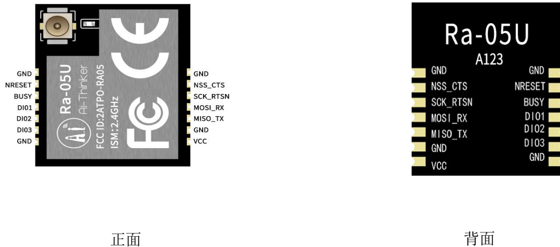
图 5 管脚示意图
