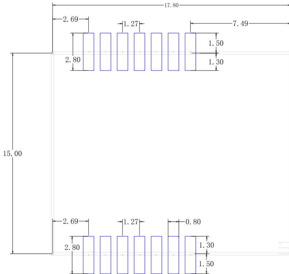
图 8 推荐 PCB 封装尺寸（单位：mm）
