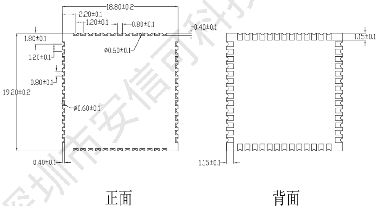
图 4 模组尺寸
