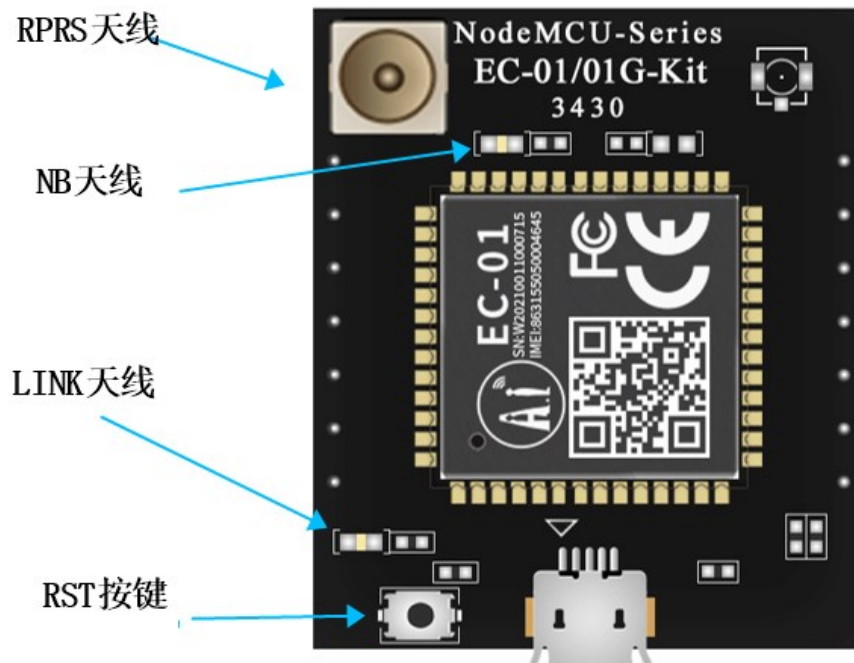
图 5 EC-01-Kit 指示灯及按键位置
