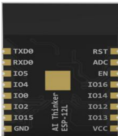
ESP-12L 管脚示意图
