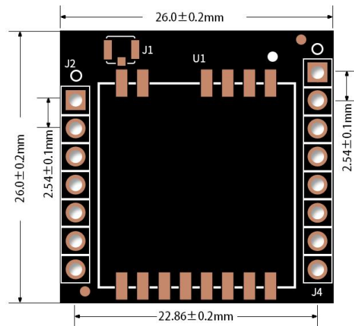
图 7 Ra-03 转接板尺寸图
