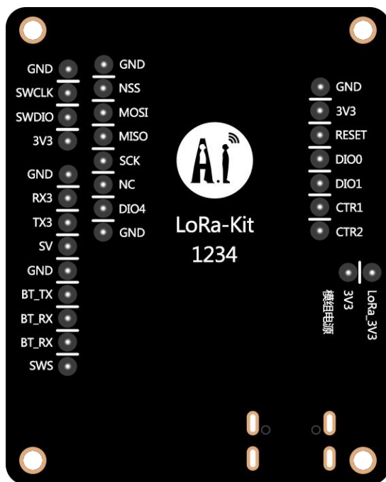
图 9 管脚示意图
