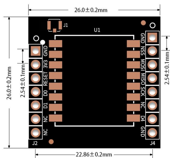
图 5 Ra-01 尺寸图
