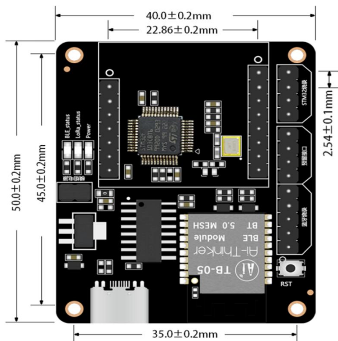
图 3 尺寸图
