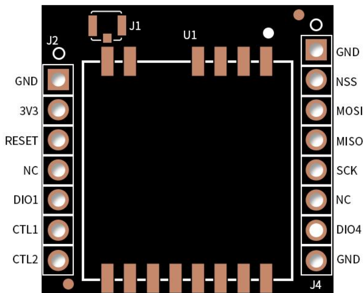
图 11 Ra-03 转接板管脚示意图
