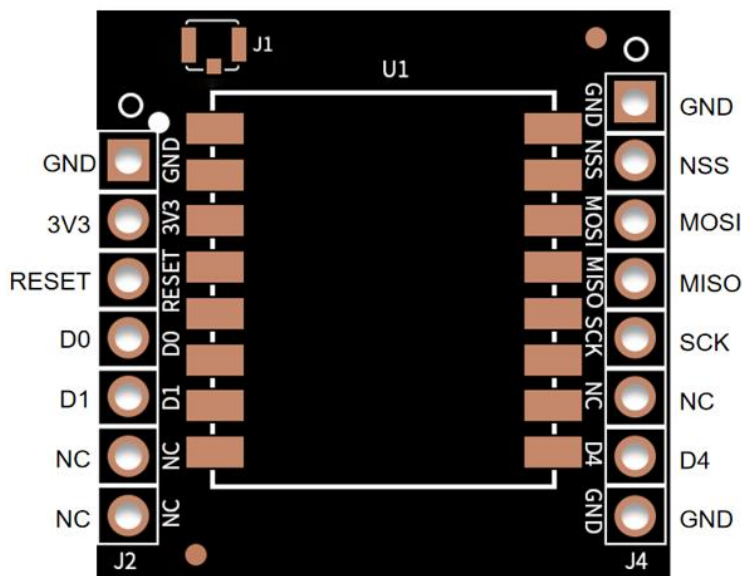
图 10 Ra-01 转接板管脚示意图
