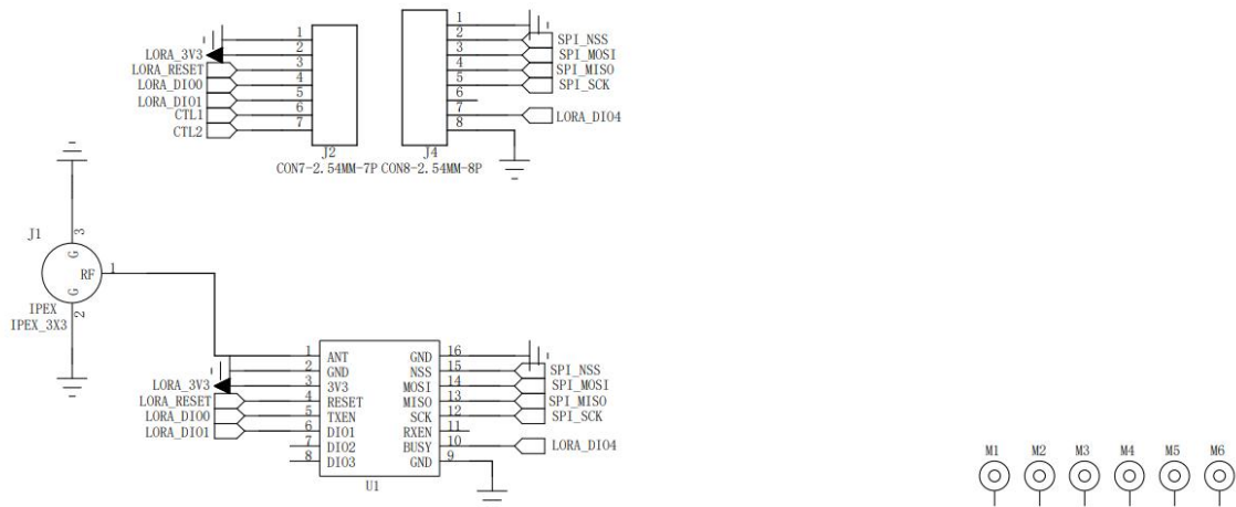
图 13 Ra-01 转接板原理图
