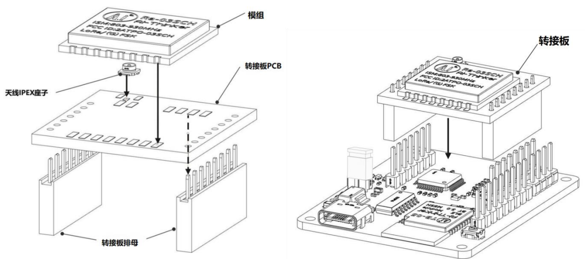
图 8 安装示意图
