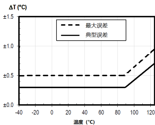
图4 GXHT30 温度误差
