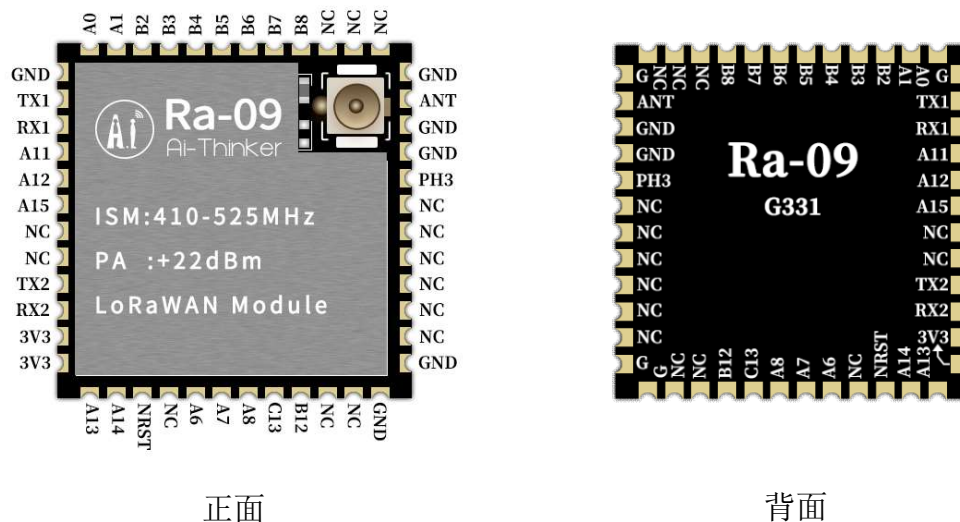
图 5 模组管脚示意图
