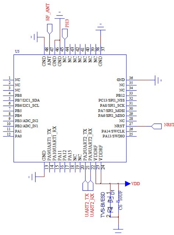
图 7 应用电路图
