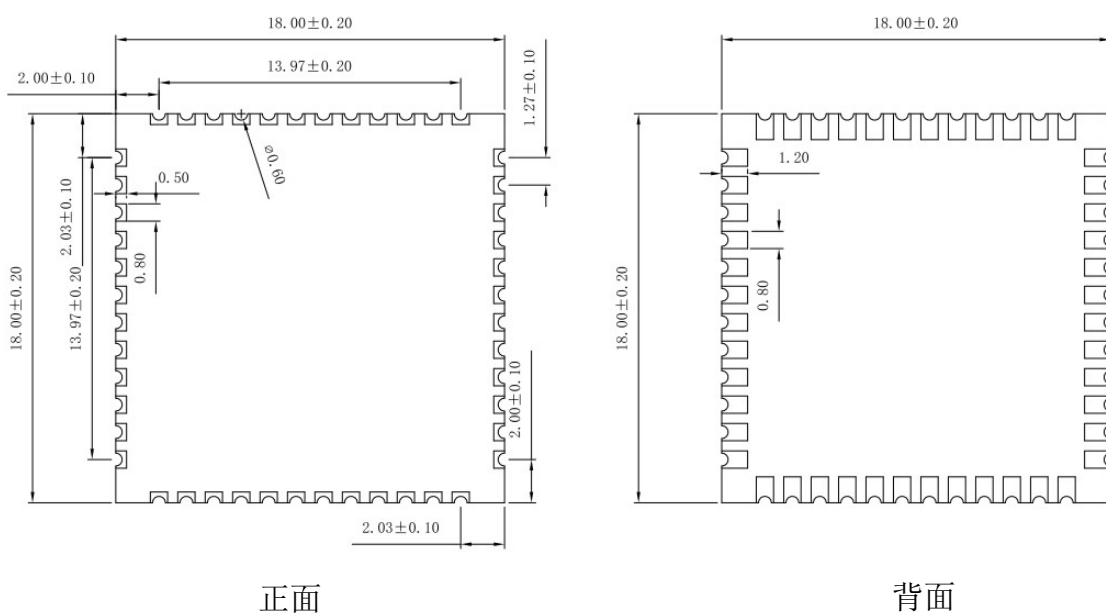
图 4 模组尺寸图
