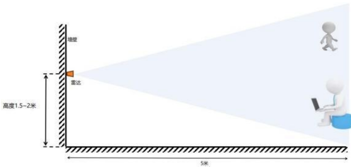
图 12 挂壁安装示意图
