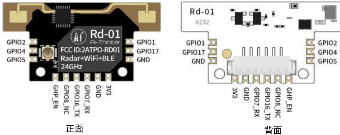
图 6 管脚示意图
