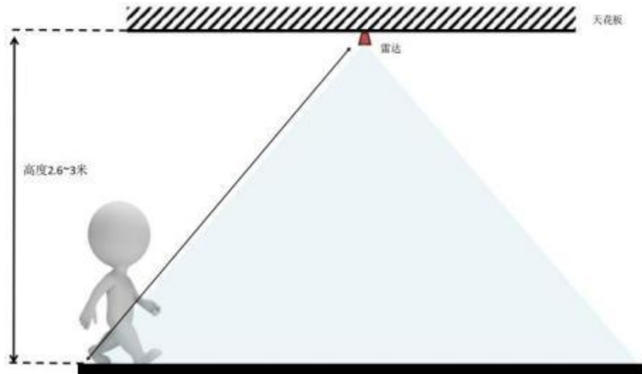
图 10 挂顶安装示意图
