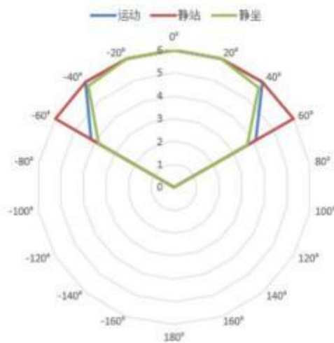
图 13 挂壁安装探测范围示意图
