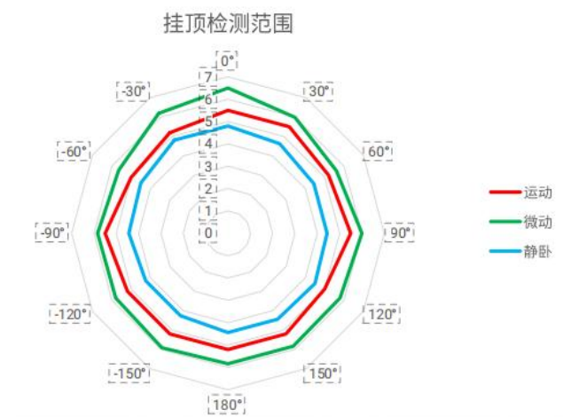
图 11 挂顶雷达图
