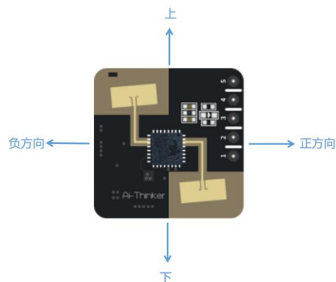
图 13 挂壁方向示意图
