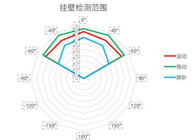
图 14 挂壁雷达图
