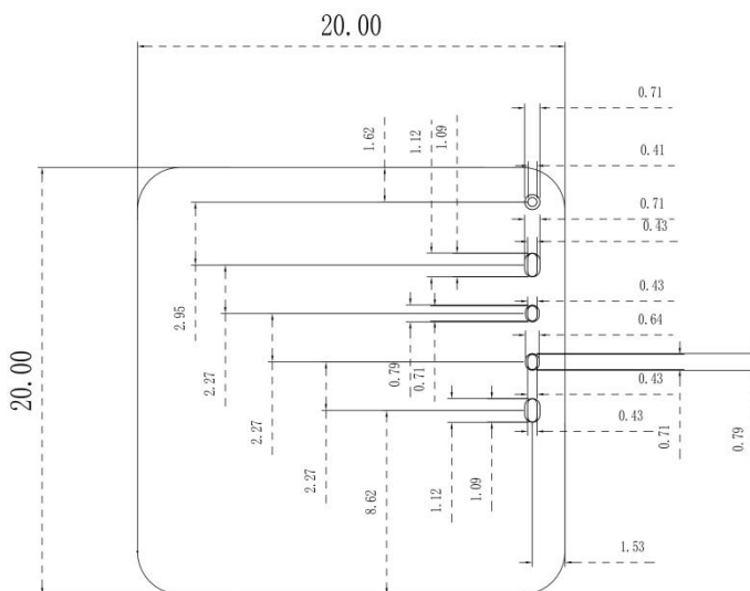
图 8 推荐 PCB 封装尺寸 (单位: mm)
