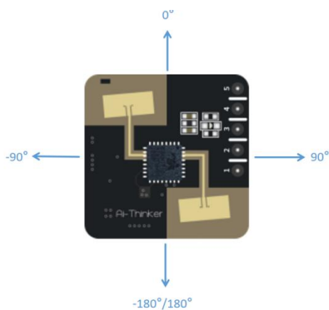
图 10 挂顶方向示意图
