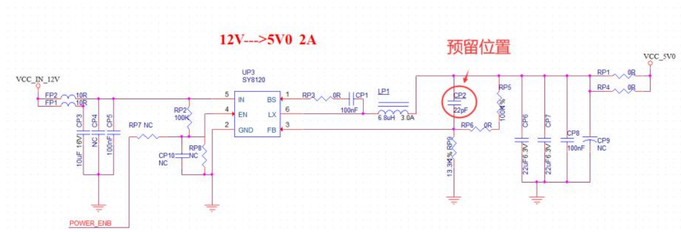
图 11 DC-DC 降压电路图
