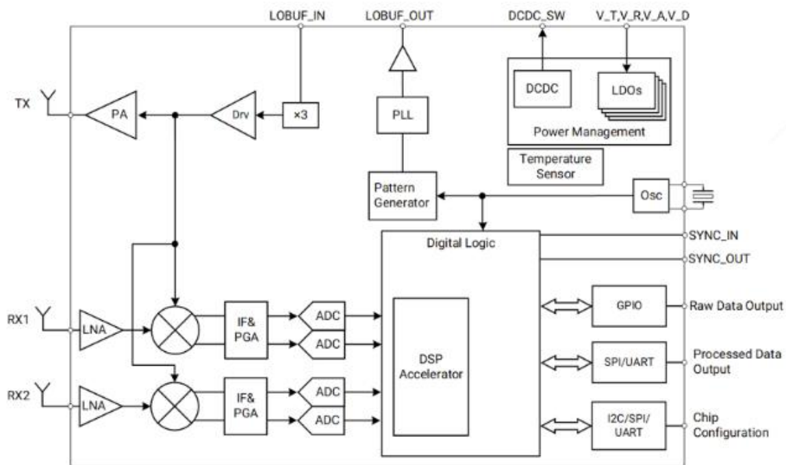
图 1 ICL1122 芯片架构图
