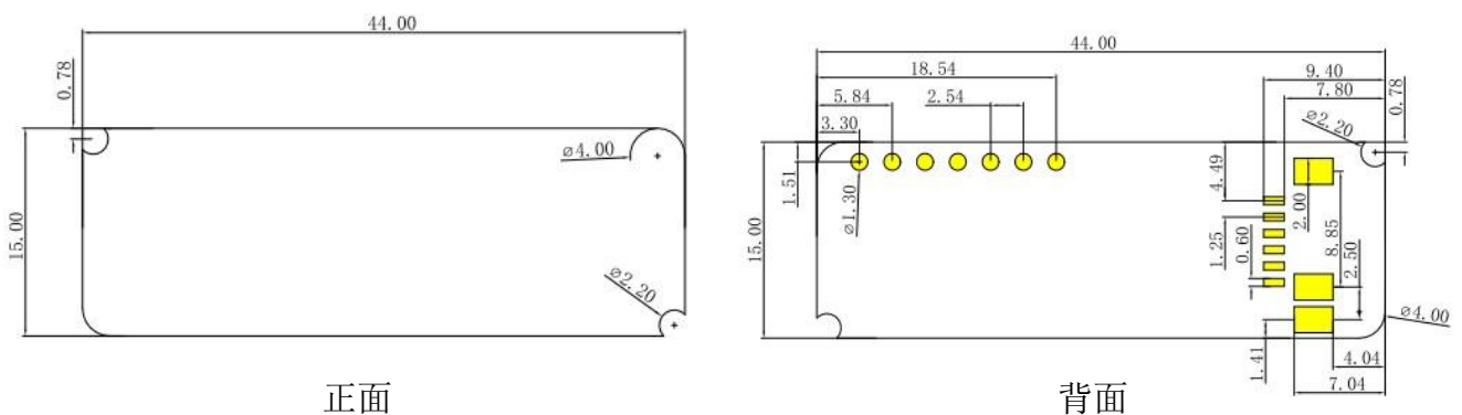
图 4 尺寸图
