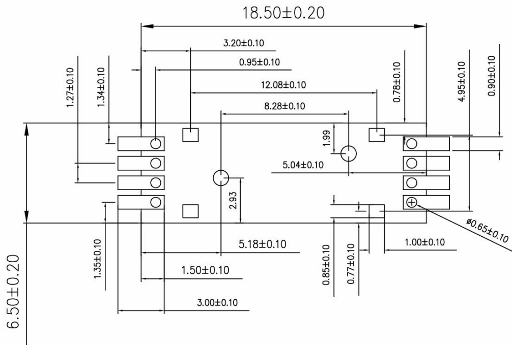
图 8 推荐 PCB 封装尺寸
