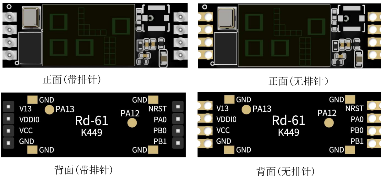
图 3 外观图（渲染图仅供参考，以实物为准）
