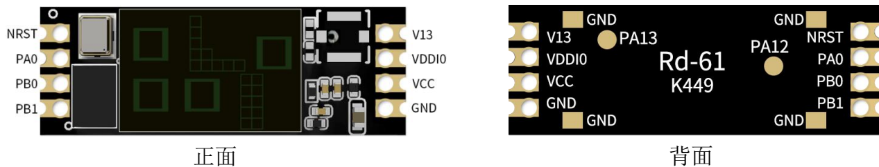
图 5 管脚示意图
