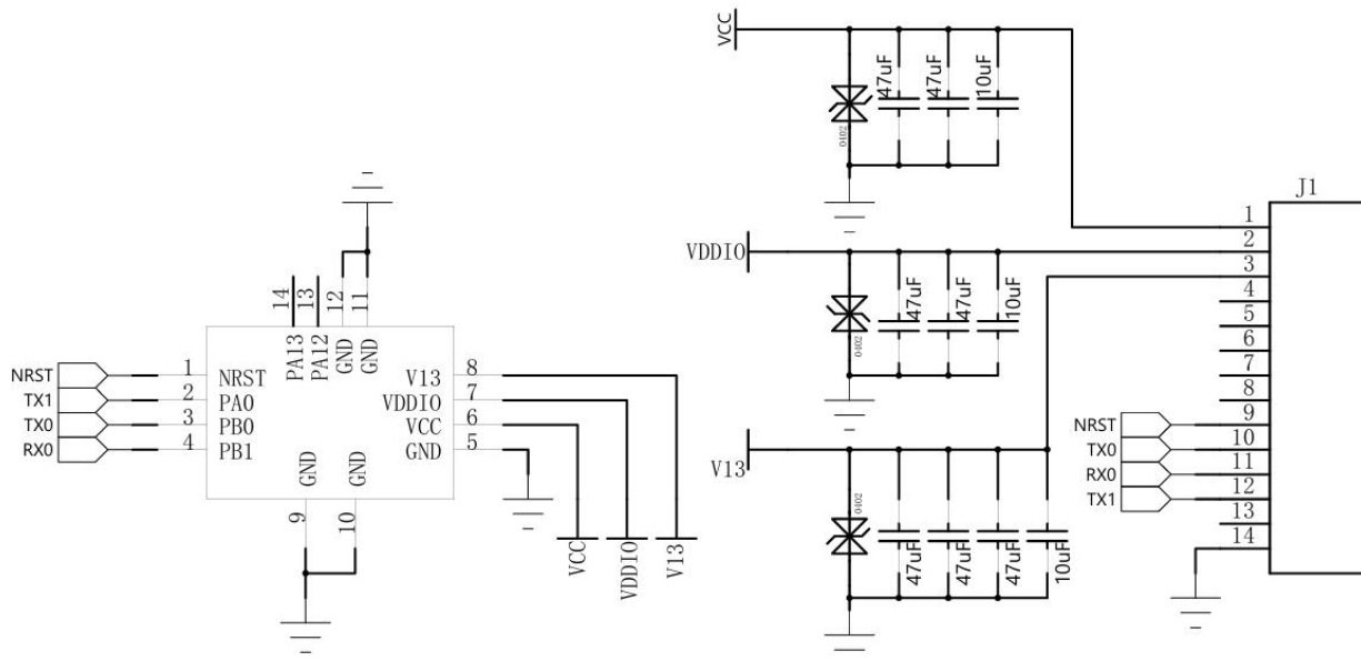
图 7 应用指导电路
