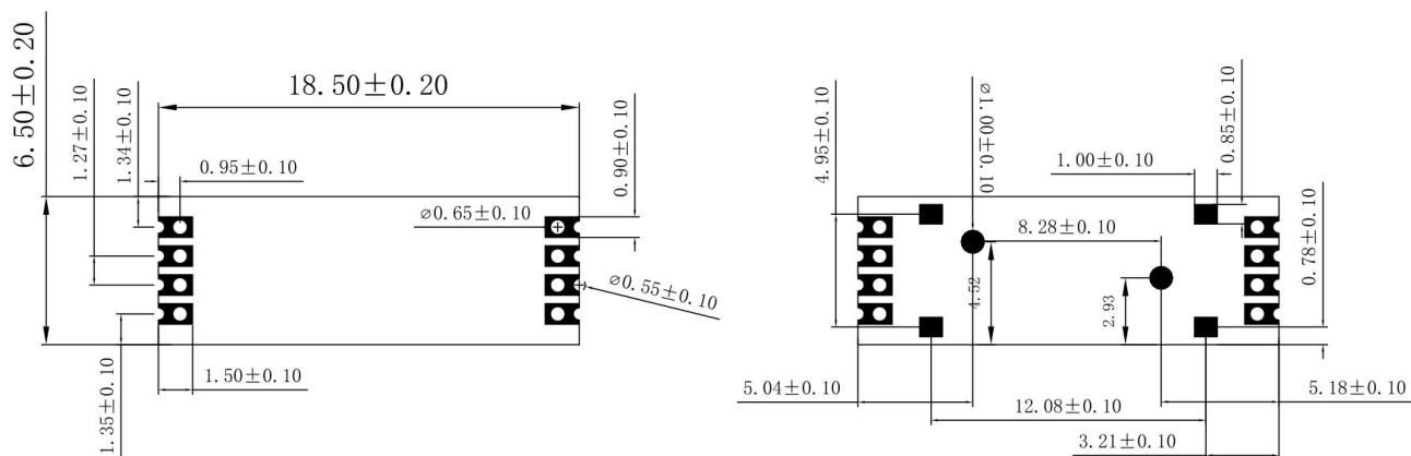
图 3 外观图（渲染图仅供参考，以实物为准）
