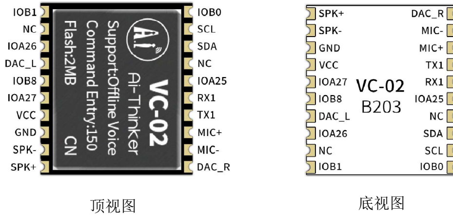
图 5 模组管脚示意图
