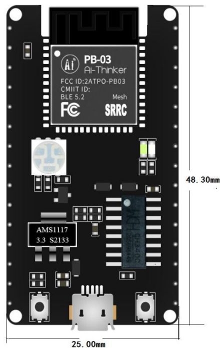
图 5 开发板尺寸图
