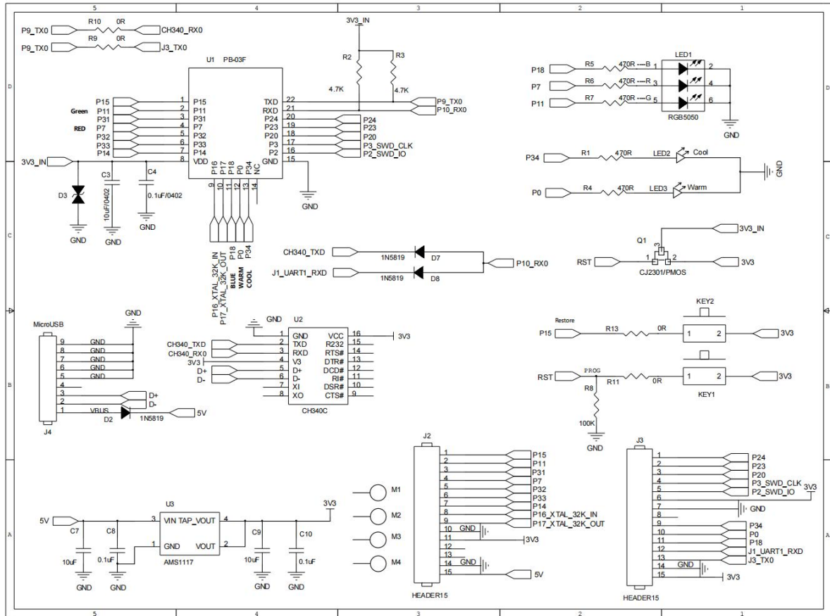
图 8 开发板原理图
