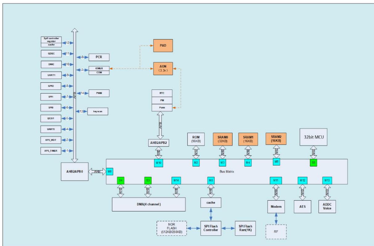
图 1 PHY6252 芯片架构图
