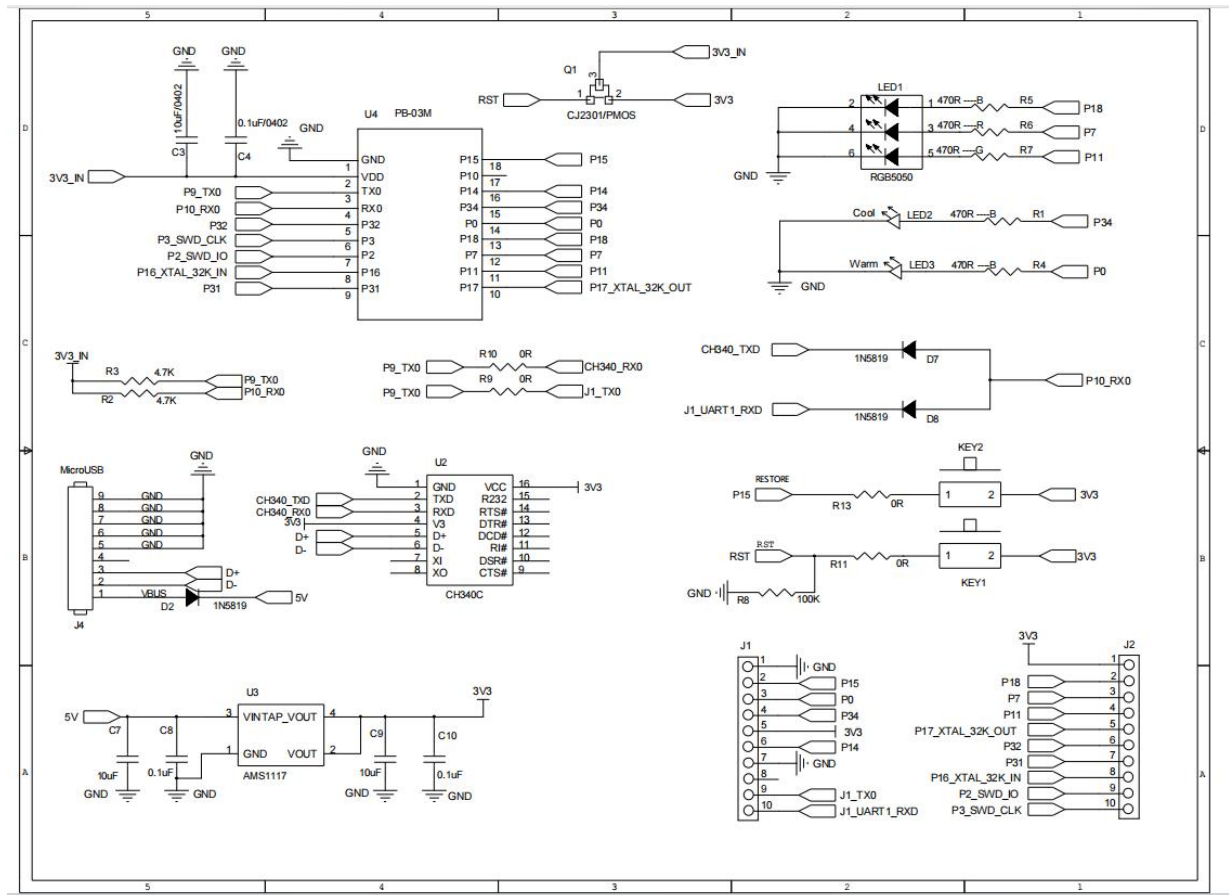
图 8 开发板原理图
