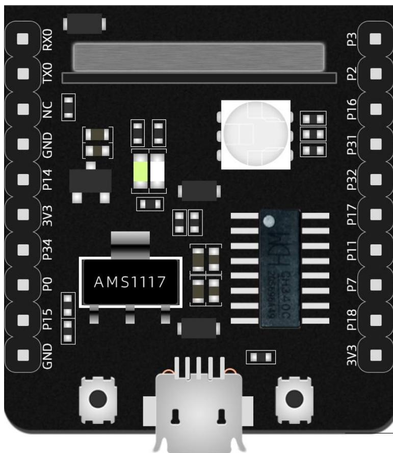
图 7 开发板管脚示意图（顶部视图）
