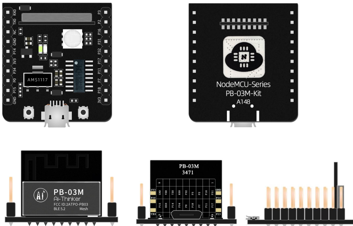
图 4 PB-03M-Kit 外观图(图片及丝印仅供参考，以实物为准)
