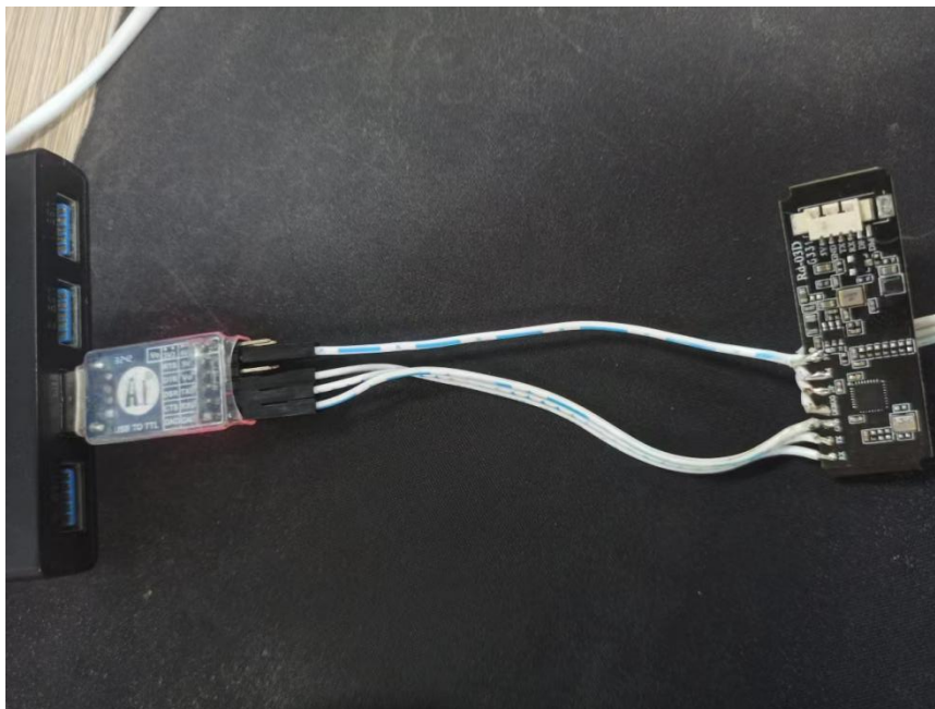
图 1.2 Rd-03D_V2 模组通过焊点与串口工具连接
