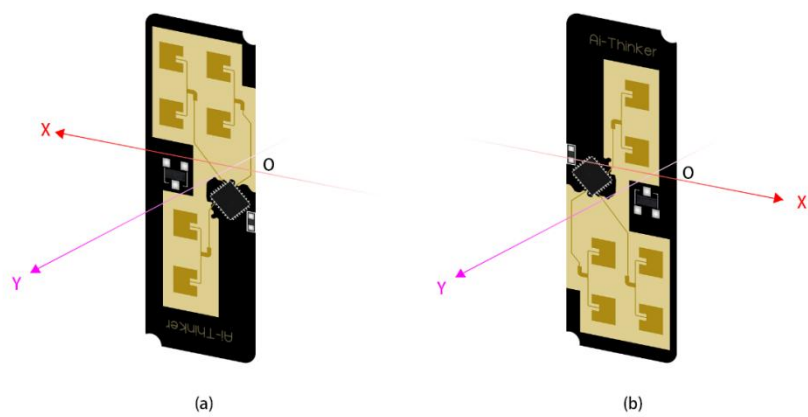
图 3-1 推荐安装方式下的目标位置坐标系示意图
