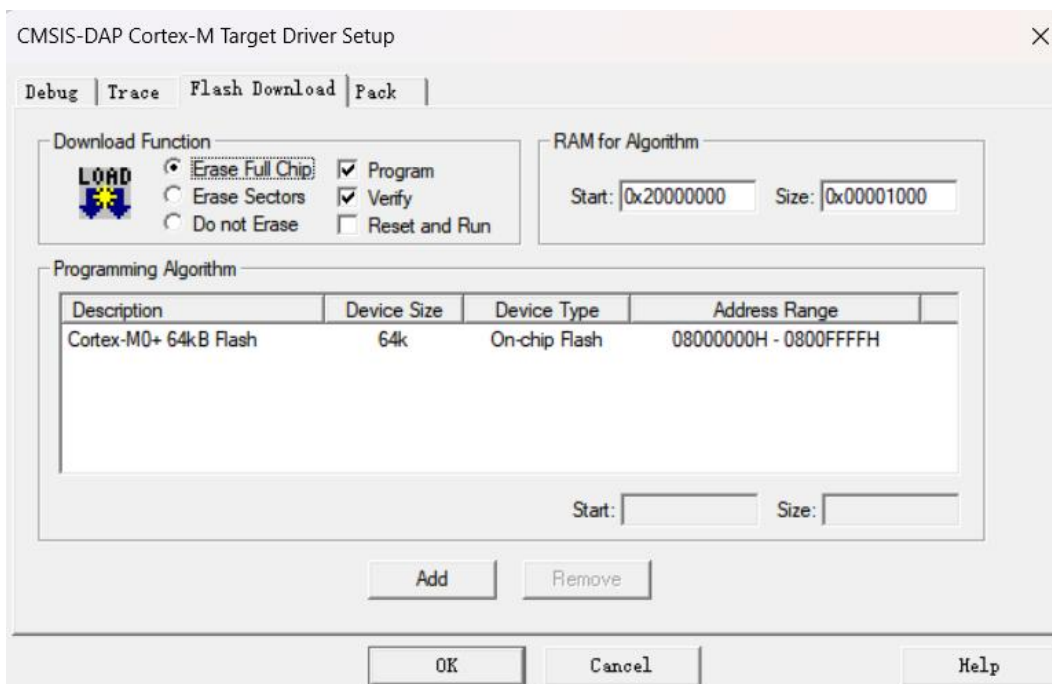
图 6. hex 文件烧录步骤 6--选择擦除 flash
