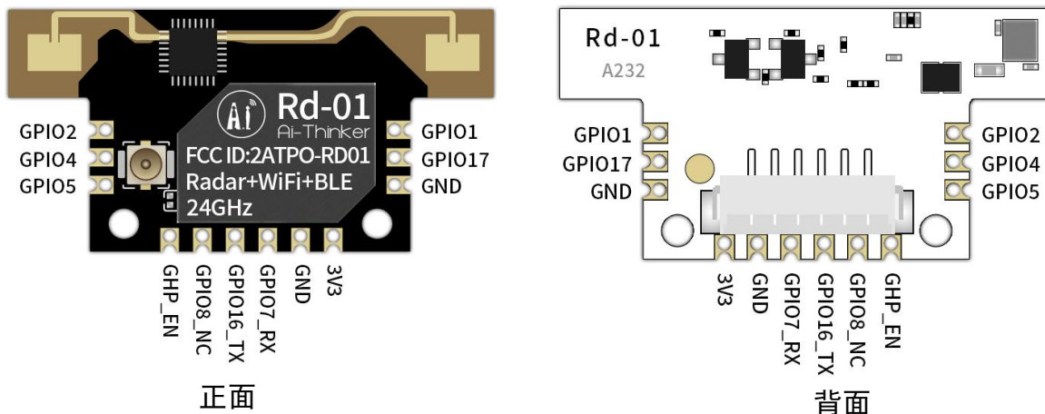
图 6 管脚示意图
