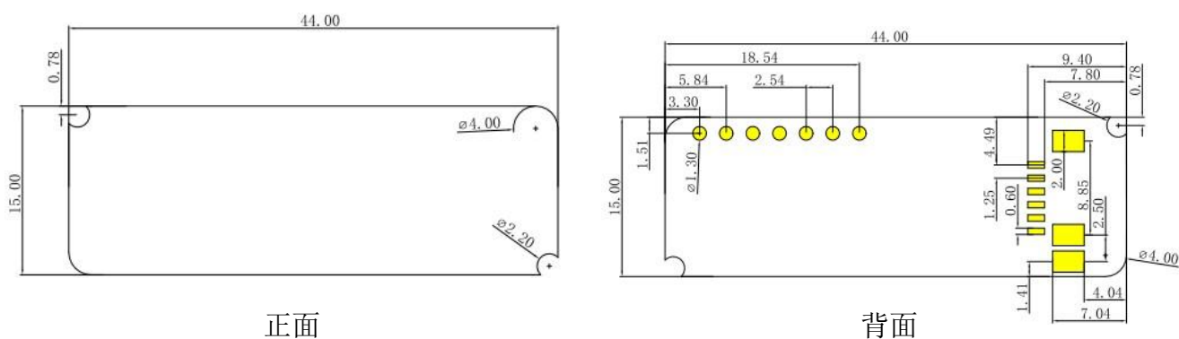
图 4 尺寸图（单位：mm）
