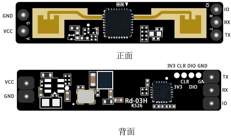
图 5 管脚示意图
