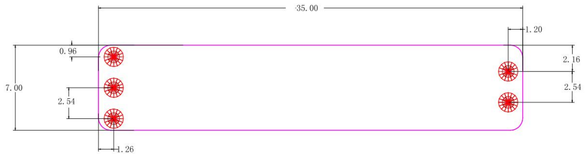
图 8 推荐 PCB 封装尺寸（单位：mm）
