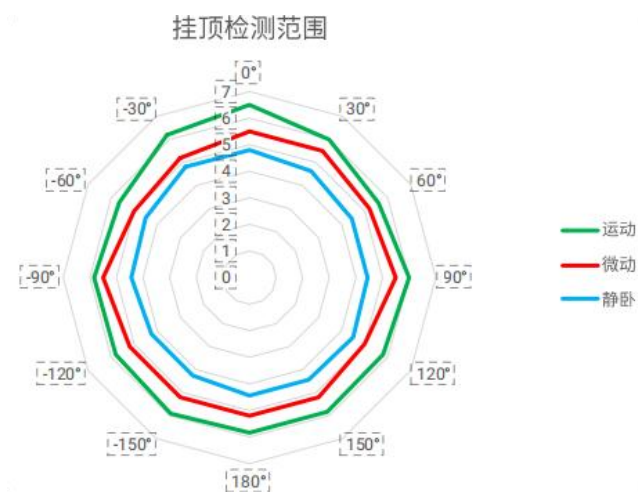
图 11 挂顶雷达图
