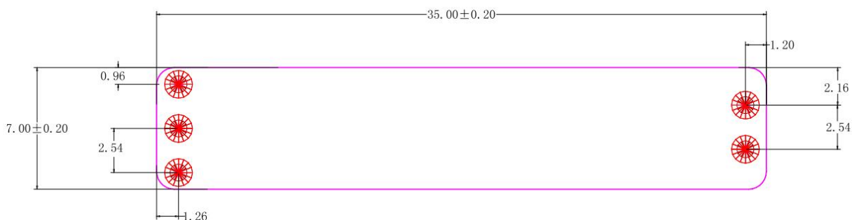
图 4 尺寸图（单位：mm）
