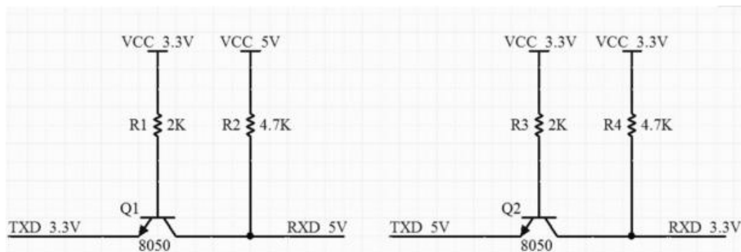
图 16 电平转换电路
