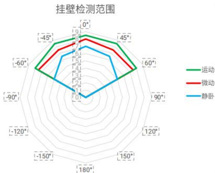
图 14 挂壁雷达图
