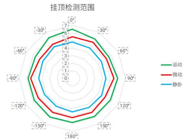
图 11 挂顶雷达图
