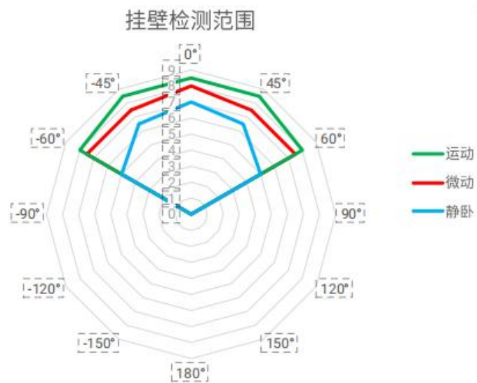
图 14 挂壁雷达图
