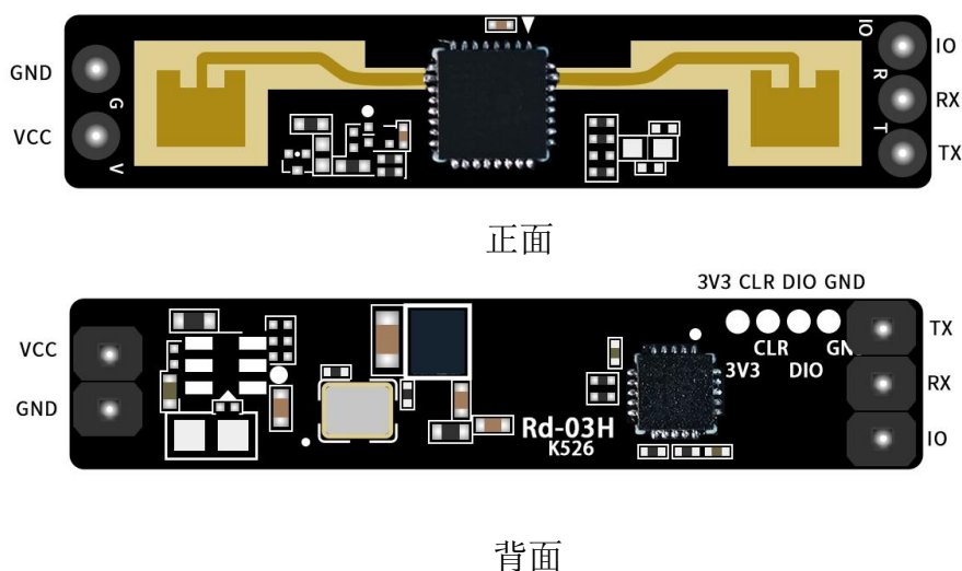
图 1 管脚示意图
