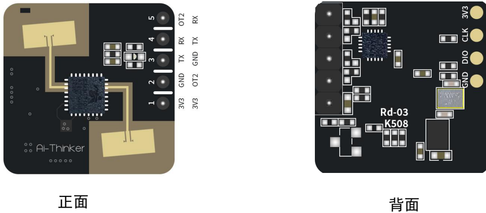
图 1 管脚示意图
