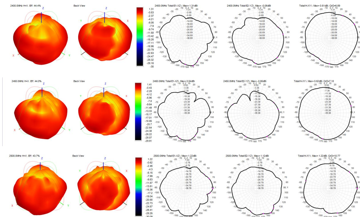
图 9 天线场型图
