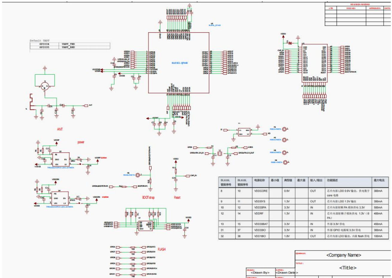
图 7 原理图
